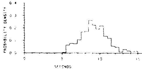
AV BENDING PERIOD, T B FULL LOAD CONDITIONS
