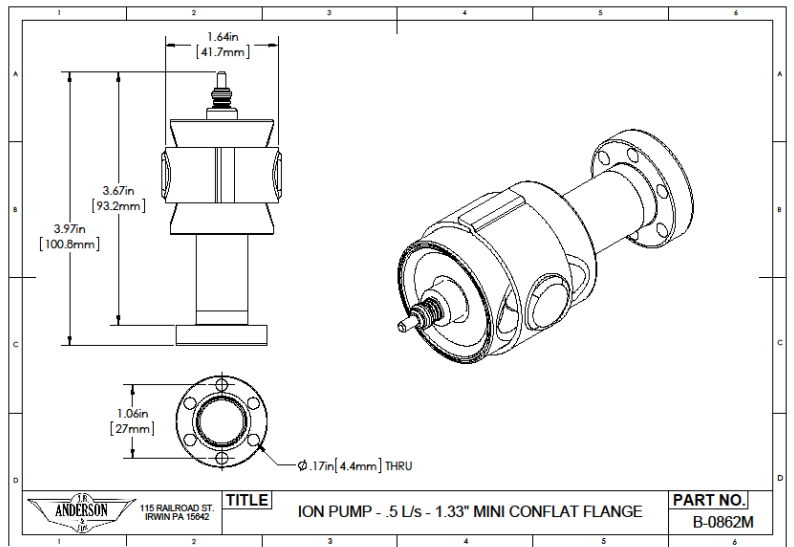
.5l/s MODION® (Mini Conflat)
