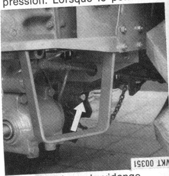
Vis magnétique de vidange
