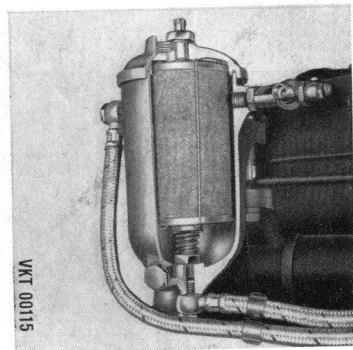
Coupe de la turbine Coupe du filtre à air à bain d'huile Coupe du filtre à carburant.
