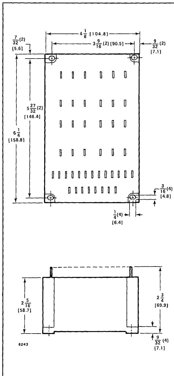
FIG. 2—MOUNTING DIMENSIONS FOR W7080A, W7081A, W7082A, W7083A, W7084A UNITS IN IN. [mm IN BRACKETS].
