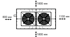
МОДЕЛИ 145 - 190 (вид сверху)
