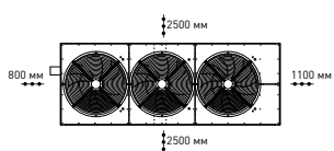
МОДЕЛИ 145 - 190 (вид сверху)
