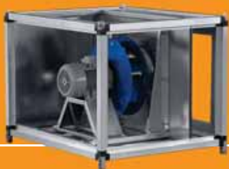
G2 – ВЫХЛОП ВВЕРХ
