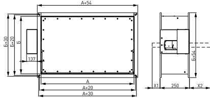
КЛАПАН С ОГНЕСТОЙКОСТЬЮ 60 И 90 МИНУТ
