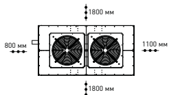
МОДЕЛИ 096 - 128 (вид сверху)
