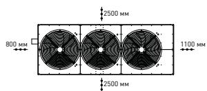
МОДЕЛИ 145 - 190 (вид сверху)
