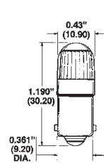
Fig. 3 Min. Bayonet Base
