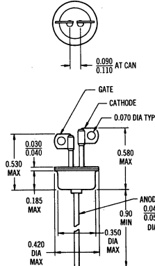
CASE 88
