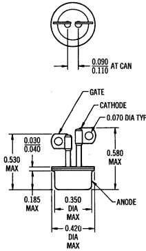
CASE 88
