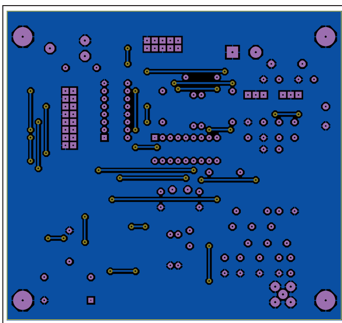
Figure 4 : Implantation du générateur côté soudures.
