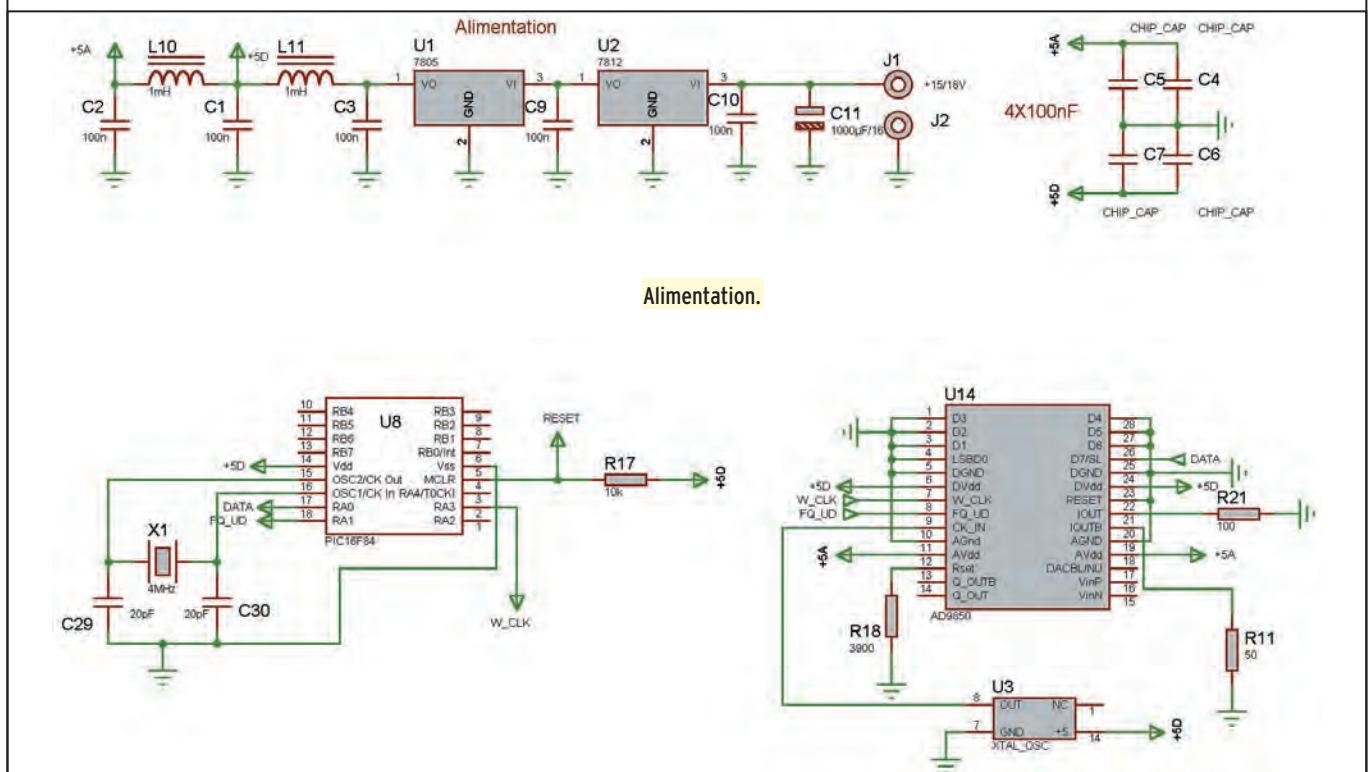
Figure 1 : schéma complet du générateur.
