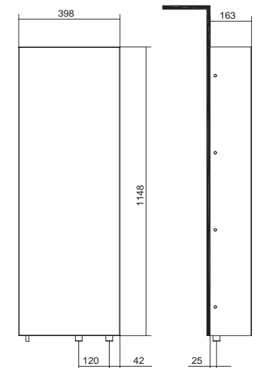
DIMENSIONS
