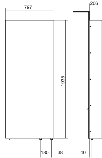
DIMENSIONS
