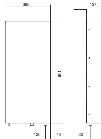
DIMENSIONS
