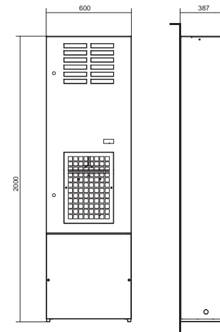
DIMENSIONS
