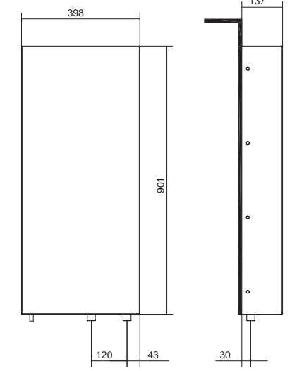
DIMENSIONS
