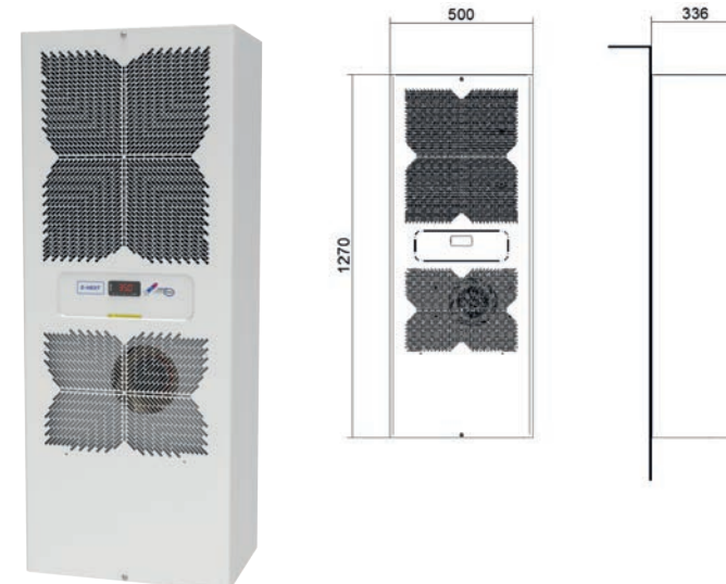
DIMENSIONS
