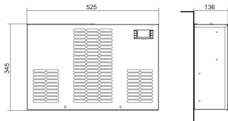
DIMENSIONS
