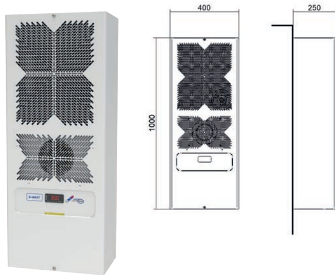
DIMENSIONS
