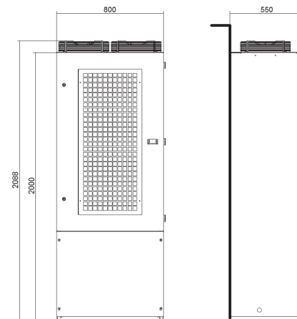
DIMENSIONS
