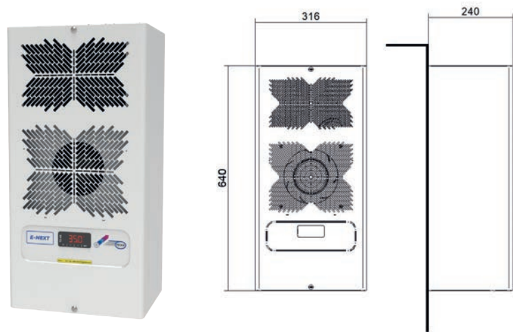
DIMENSIONS
