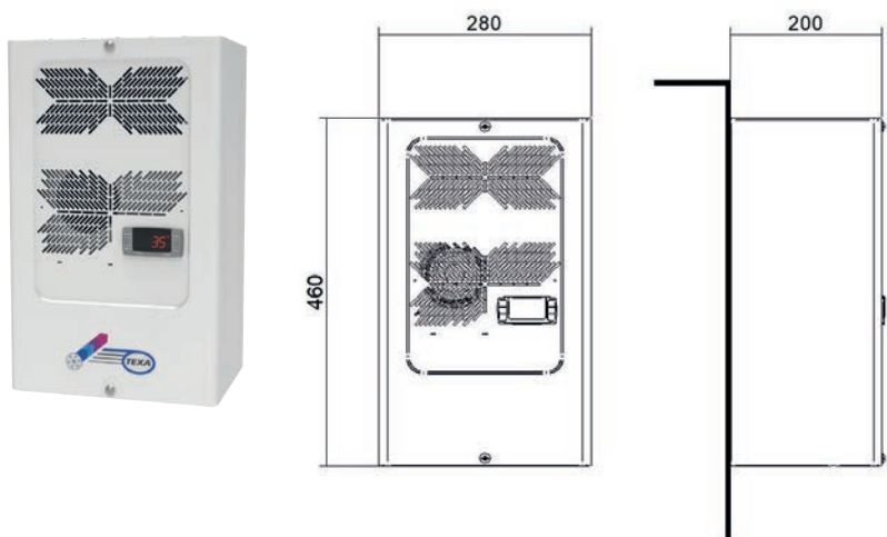
DIMENSIONS
