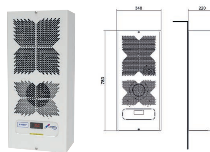
DIMENSIONS
