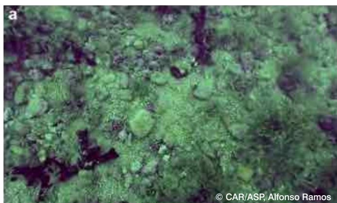
Figure 4-20. Détritique côtier avec rhodolithes : a) Arthrocladia villosa et une démosponge noire (NE-Rachgoun, -27 m) ; b) graviers recouverts de Corallinales encroûtantes (N-Rachgoun, -30 m).
