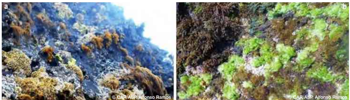
Figure 4-4. Roche médiolittorale dans le secteur Nord : a) association à Lithophyllum byssoides (taches blanches), et association à Nematolium helminthoides (algue filamenteuse marron) et Rissoella verruculosa (tâches orangées) ; b) associations à Ceramium ciliatum et à Gelidium pusillum (tâches marrons), avec la chlorophyte Ulva rigida (tâches vertes) et Cystoseira amentacea (tâche marron obscure en haut à la gauche).
