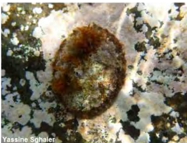
Figure 7-16. Patella safiana dans le secteur sud de Rachgoun à -1 m.
