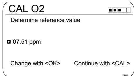
Fig. 76: Reference value
