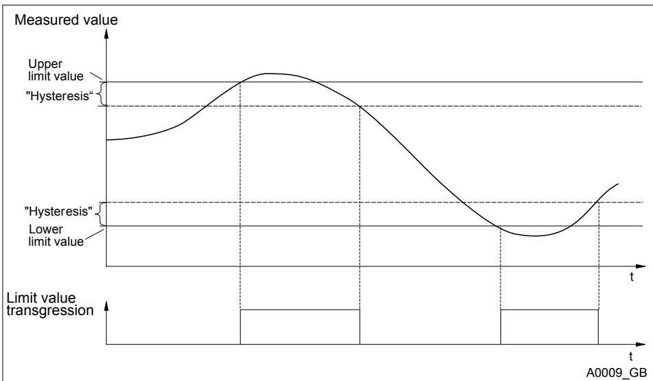
Fig. 96: Hysteresis
