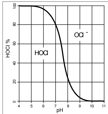
Fig. 35: HOCl/OCl equilibrium
