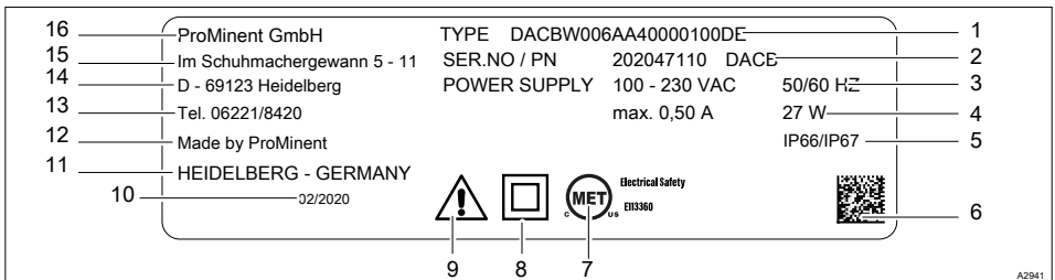
Fig. 10: Nameplate, MET
