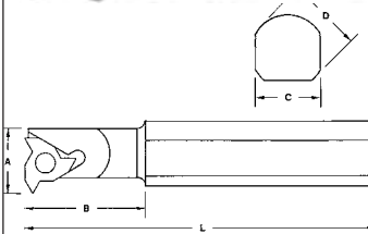
AT-1V V-Holder
