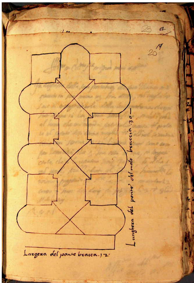
Disegno del ponte del molo di Livorno, 1567 ottobre 1, f. 532, c. 20.
