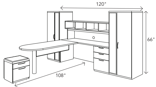
PO.L 013 120W 108+D 66H
