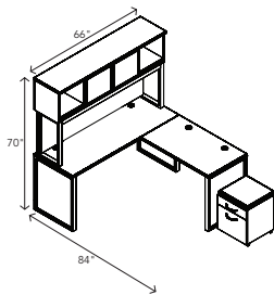
SH.L.008 66W 84+D 70H
