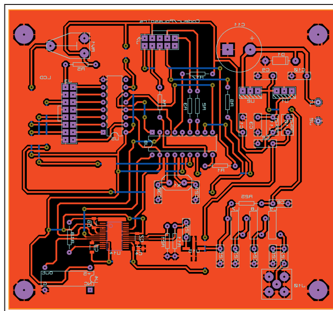
Figure 2 : Circuit imprimé du générateur.
