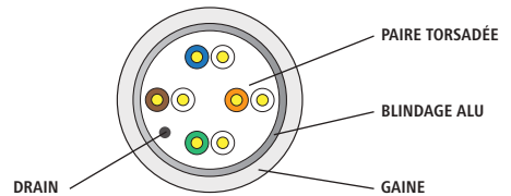
F/UTP
