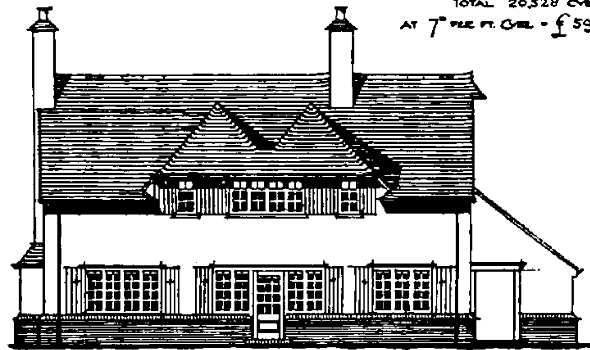
• S.E. ELEVATION •
