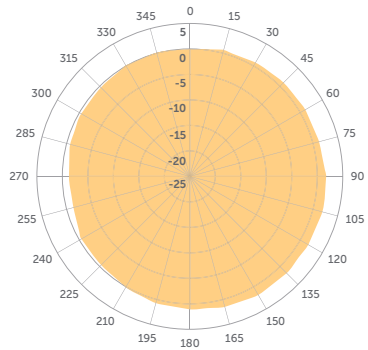
5 GHz Horizontal
