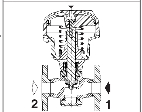
NO function
