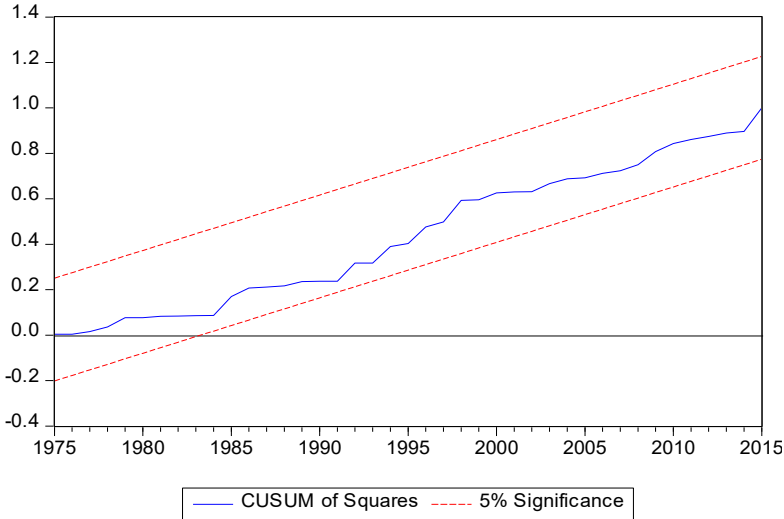
Şekil 2. CUSUM ve CUSUMSQ Grafikleri
