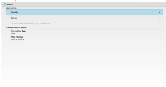
5) Страница Ethernet
