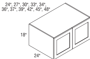
W241824-W371824 Butt doors W391824-W481824CS Center mullion
