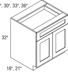
VB2432 __-VB3632 __ Butt doors
