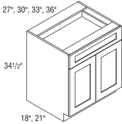
VB2434 -VB3634 - Butt doors
