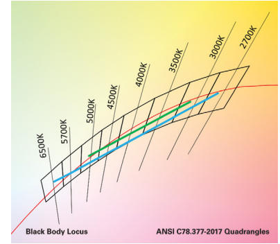
3000K - 5000K 2700K - 6500K
