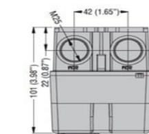
Maatschets 60-SM1Z1701P met noodstop
