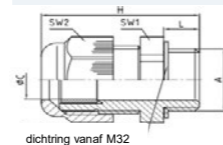
dichting vanaf M32
