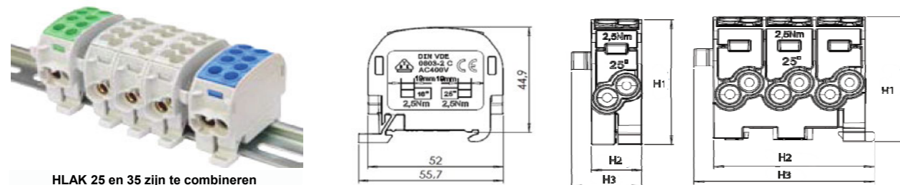
HLAK 25 en 35 zijn te combineren
