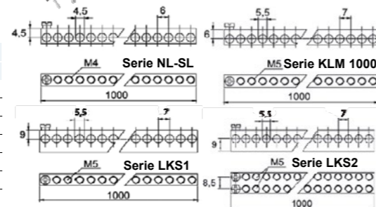
Serie LKS2
