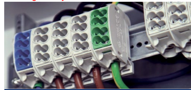
HORA Etec klemmen, veilig en gebruiksvriendelijk!
