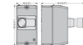
Maatschets 60-SM1Z1701P met noodstop
