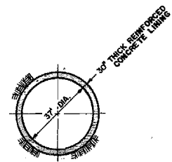
SECTION E-E SCALE: B
