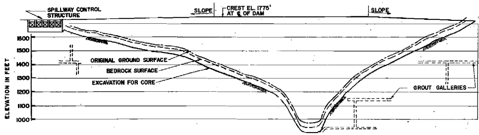
LONGITUDINAL SECTION THRU & OF DAM SCALE: B
