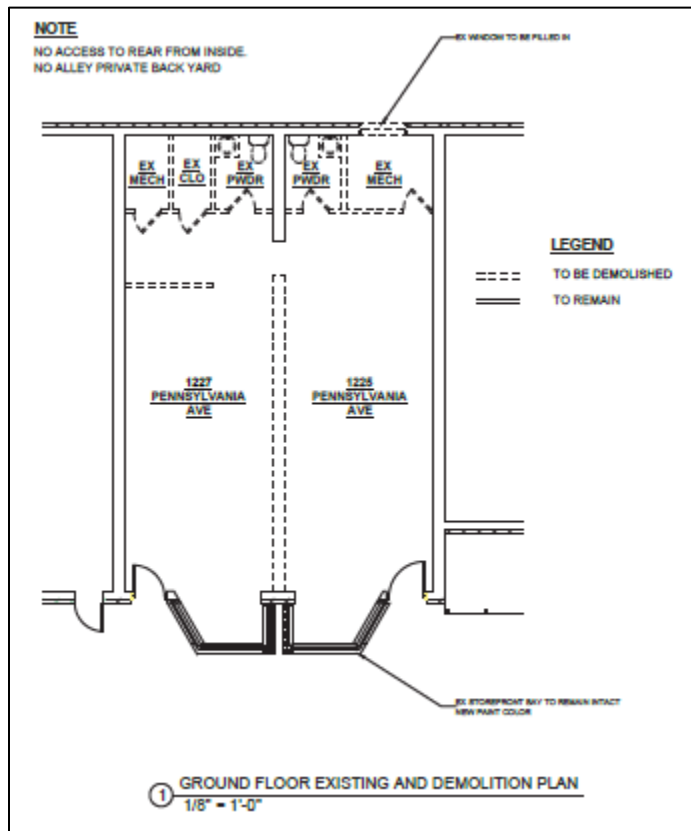
Plan d'étage de 1225/1227 PENNSYLVANIA AVE. SE, Washington, DC. En 2018.
