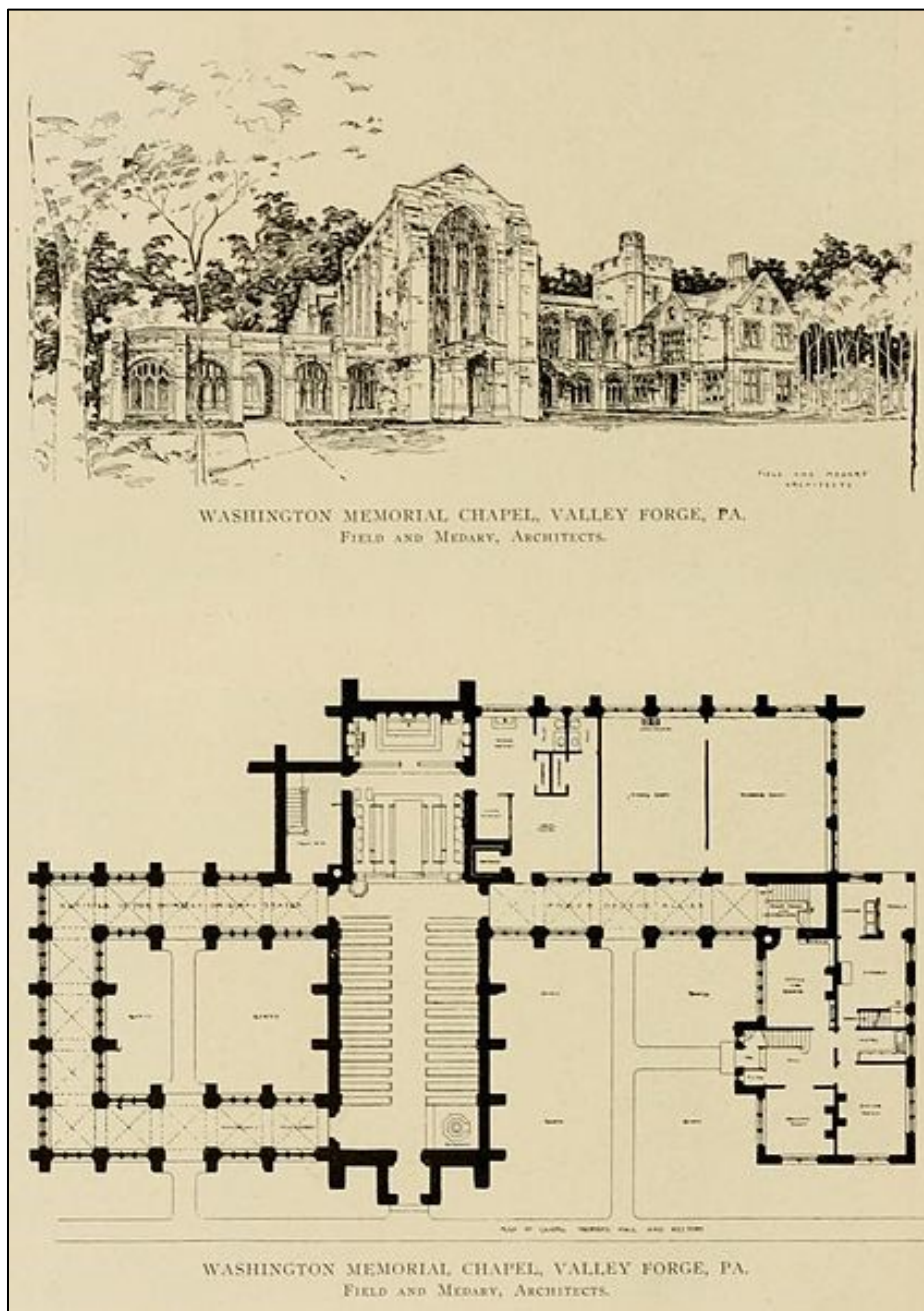
Plan d'étage original de la Washington Memorial Chapel à Valley Forge.
