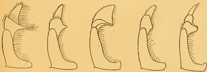
a. rupestris
