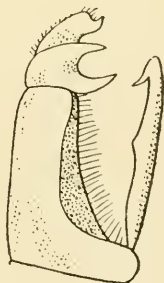
14 pomorum
