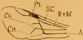
Fig. 7 — Cleptes sp. fortement grossi (d'après BUISSON), figure empruntée à HANDLIRSCH.
