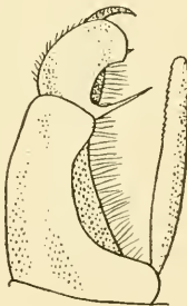
10 agrorum
