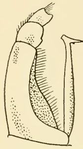
7 lapidarius
