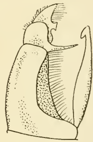
12 silvarum
