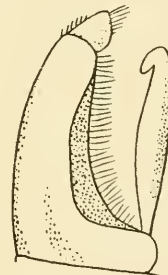
11 hypnorum
