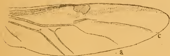
Fig. 5. — Aile d' Apatetica (d'après BONDROIT).
