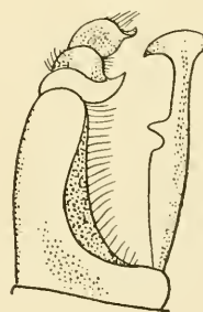
15 Latreillellus
