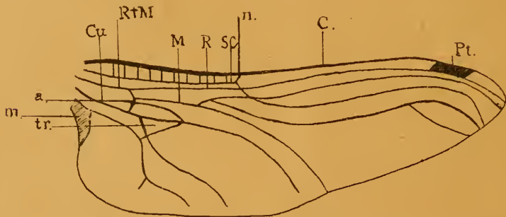
Fig. 1. — Eschna affinis VANDERL. 2/1 (aile postérieure) d'après K. REZSÖ. C = costale, sc = sous-costale. R = radiale, M = médiane, Cu = cubitale, a = arculus, n = nodus, m = membranula, tr = triangle, Pt = pterostigma.
