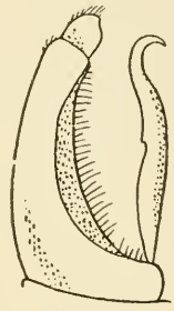
4 pratorum
