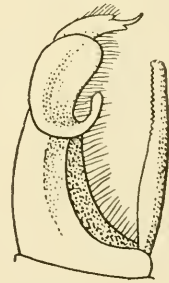
16 hortorum
