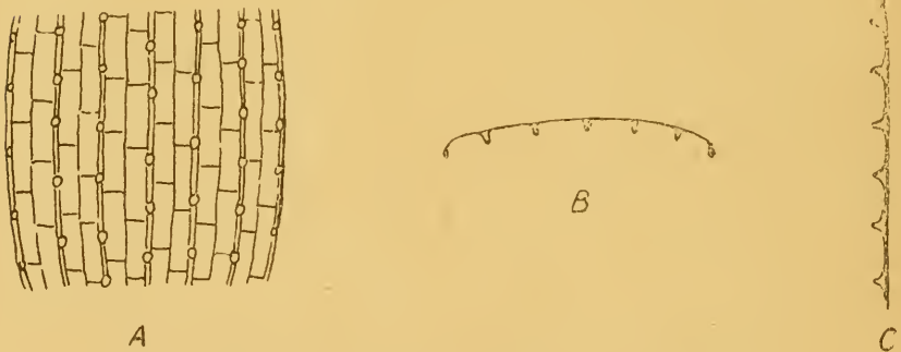
Détails de l'androconium* de Lycaena icarus . \times 2000
