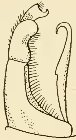
3 soroensis
