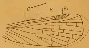
Fig. 6. — Orthophlebioides reticulatus HANDL. \times 55 — Lias d'après A. HANDLIRSCH (montre que le pterostigma dépend de la radiale).
