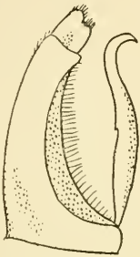
5 jonellus
