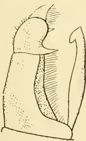
13 helferanus
