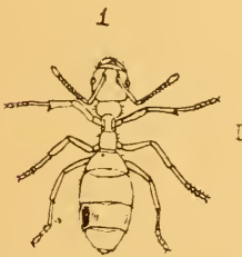
Fig. 1. Prenolepis Sakuræ ♀.
