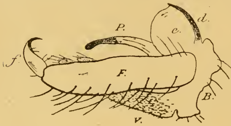
Fig. 2. — Armure génitale du mâle, vue du côté droit; \times 200 .
