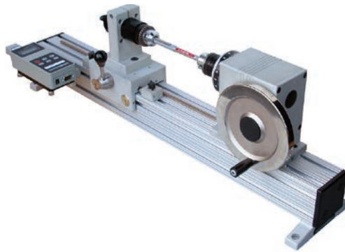
TST Test Stand Horizontal
