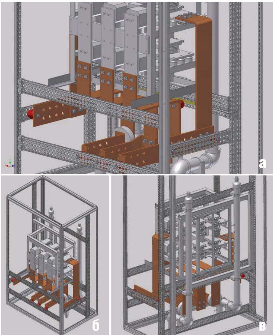
Силовой шкаф вентиляционной секции (реконструкция главных приводов стана 1300, 000 «ВИЗ-Сталь»): а — подвод шин; б — общий вид шкафа; в — система водяного охлаждения
