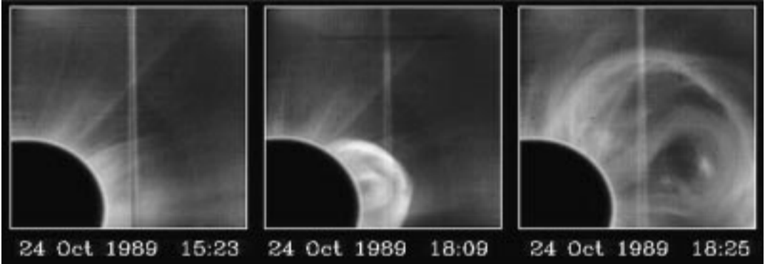
Prises lors du maximum d'activité solaire de 1989, ces photos montrent le développement rapide d'une éjection de masse coronale. Au bout de trois heures, la bulle de particules est plus grosse que le Soleil, dont le disque est masqué afin d'observer les détails de la couronne.
