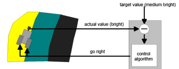
Boucle de régulation
