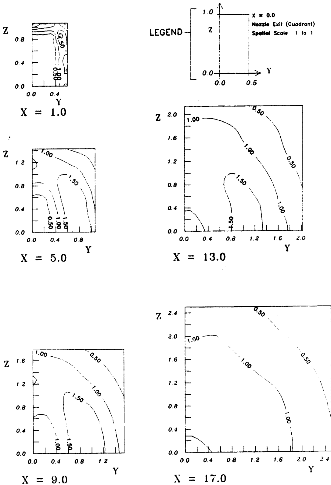
Fig. 23 1x2 Nozzle M=0.09 w_w/(U_e U_e) \times 100
