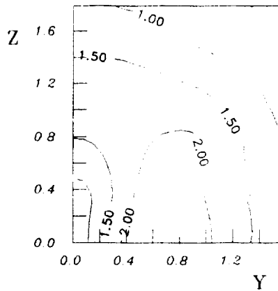
Fig. 61 1x2 Nozzle M=0.9 uu/(UeUe) \times 100
