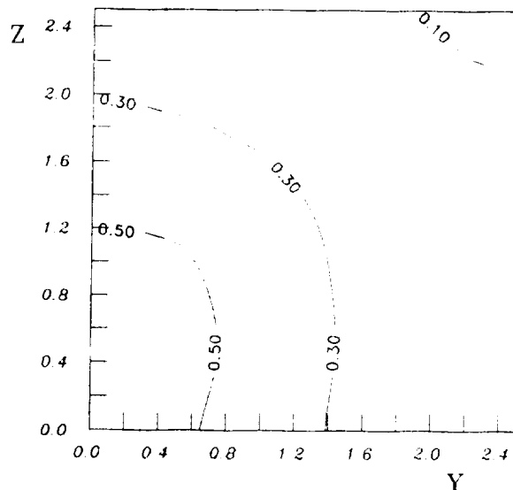
Fig. 58 M=0.9 1x2 Nozzle U/u_e
