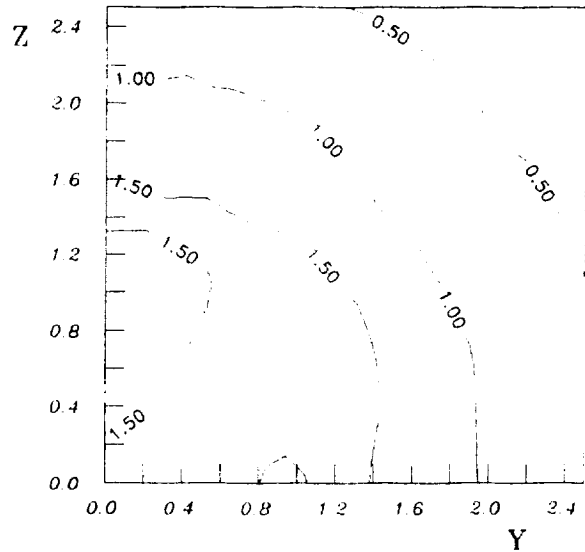
Fig. 61 1x2 Nozzle M=0.9 uu/(UeUe) \times 100
