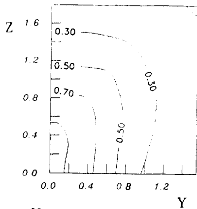
Fig. 58 M=0.9 1x2 Nozzle U/u_e
