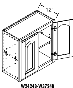
W2424B-W3724B
