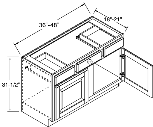
VBB3618-VBB4818 VBB36-VBB48
