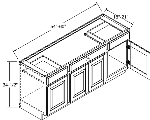
VBB5418BH-VBB6018BH VBB54BH-VBB60BH
