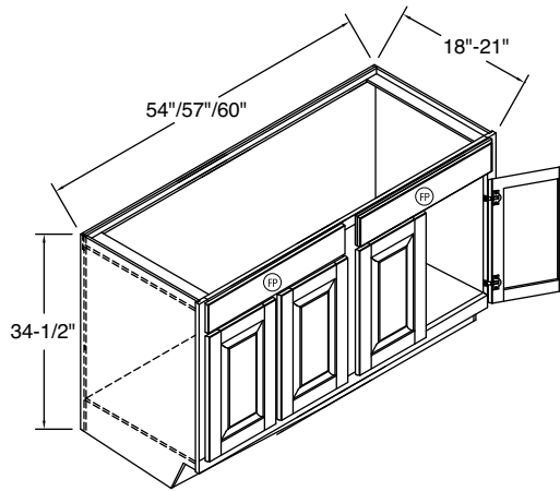
VSB5418BH-VSB6018BH VSB54BH-VSB60BH
