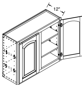
W3930-W4830
