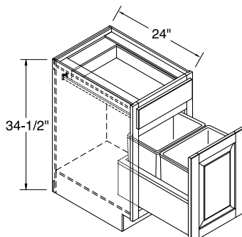
BWB18-BWB21
