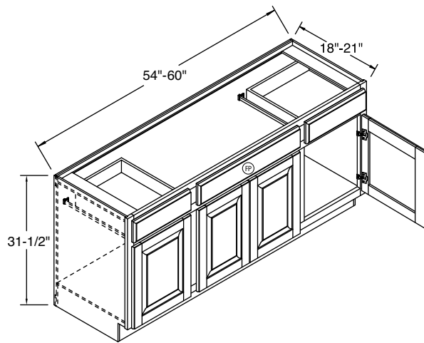
VBB5418-VBB6018 VBB54-VBB60
