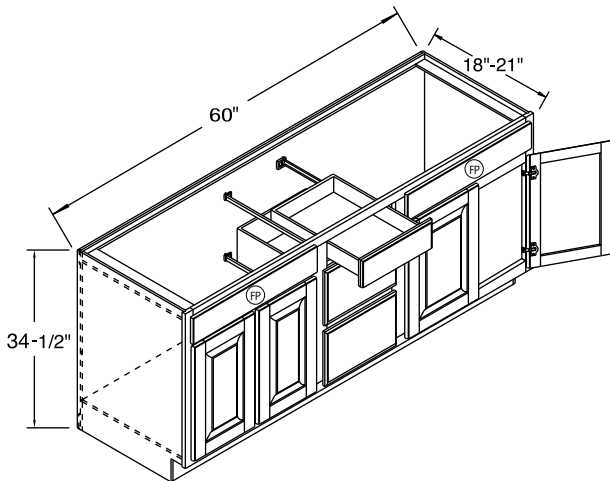
VDB6018BH-VDB60BH
