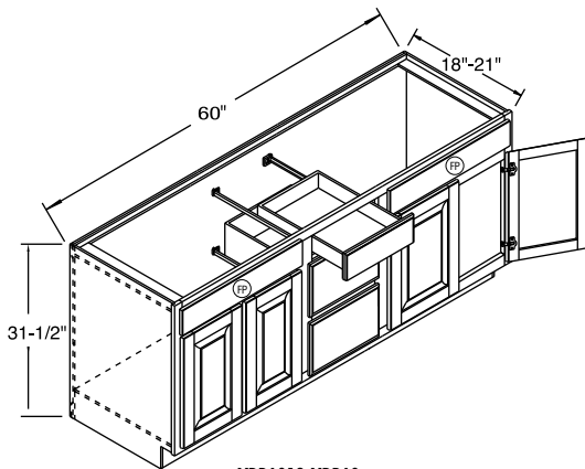
VDB6018-VDB60
