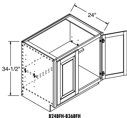
B24BFH-B36BFH
