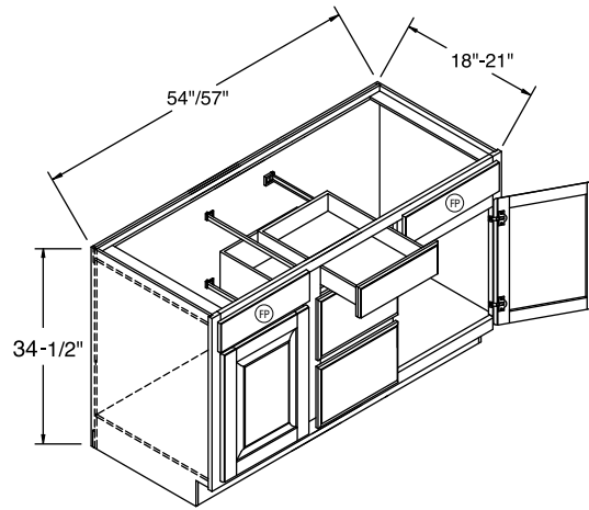
VDB5418BH-VDB5718BH VDB54BH -VDB57BH
