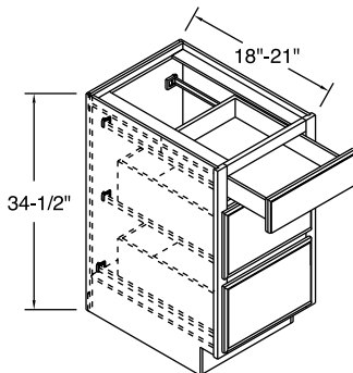
VBD1218BH-VBD2418BH VBD12BH-VBD24BH
