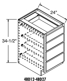
4BD12-4BD27
