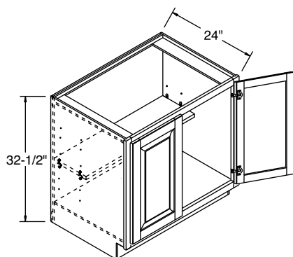
B24BFH32.5-B36BFH32.5
