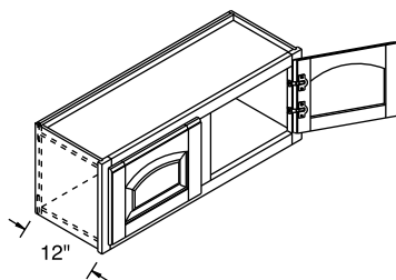
W3915
