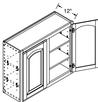
W3933-W4833
