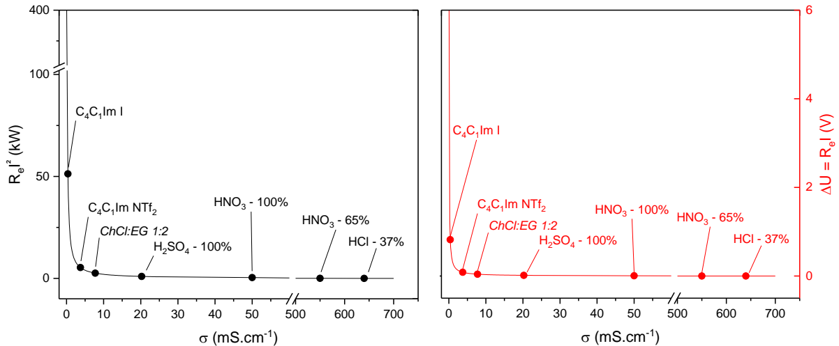
Figure III-16 - Puissance dissipée par effet Joule (gauche noir) et chute ohmique associée (droite rouge) dans l'exemple ci-dessus en fonction de la conductivité ionique de l'électrolyte
