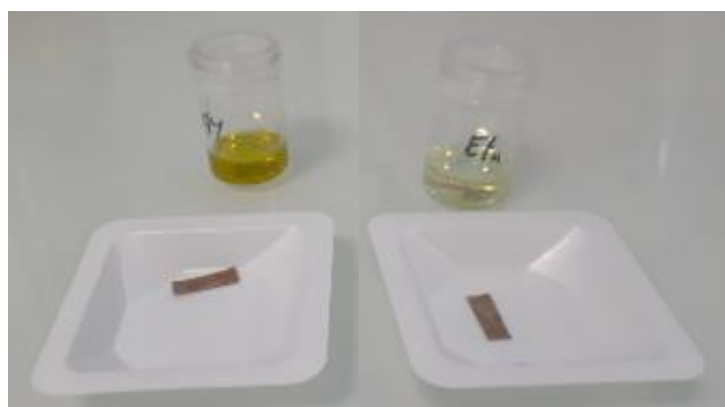
Figure IV-15 - Dissolution chimique d'une plaque de cuivre (24 h et 40 °C) dans C_4C_1Im(NTf_2)_{0,78}Cl_{0,22} (gauche) et dans ChCl:EG 1:2 (droite)
