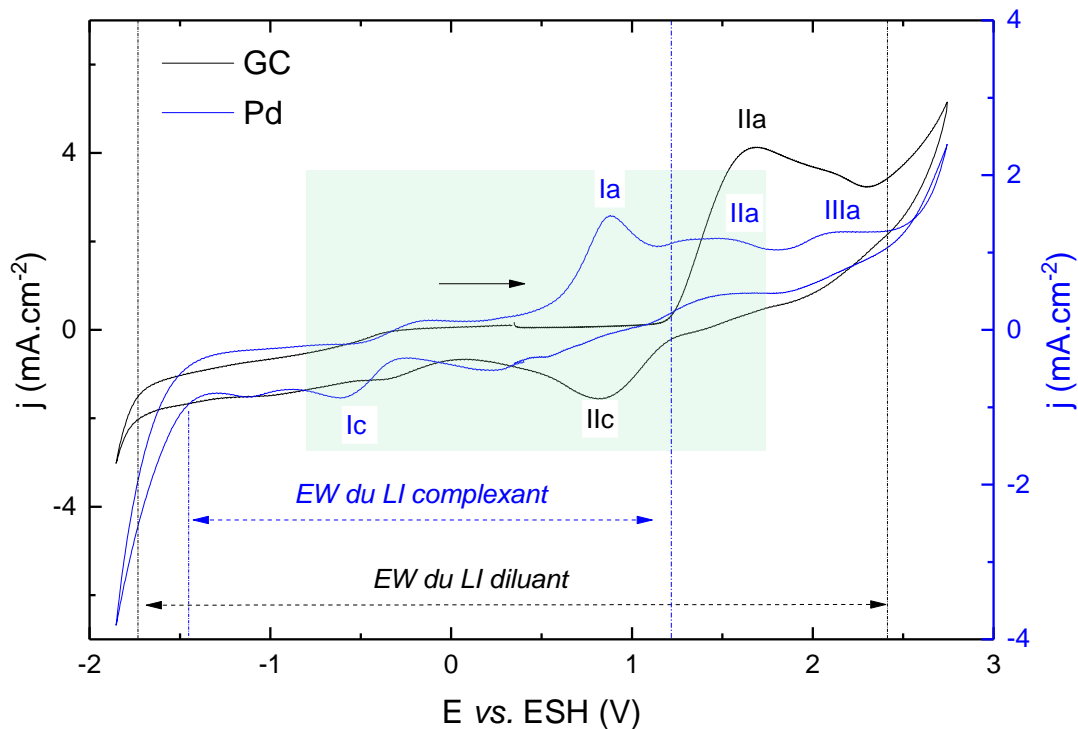
Figure II-34 - Voltampérogrammes cycliques à 50 \text{ mV}\cdot\text{s}^{-1} obtenus sur électrode de palladium (bleu) et de carbone vitreux (noir) dans C_4C_1Im (NTf_2)_{0,97}Cl_{0,03} - T = 40 \text{ }^\circ\text{C}
