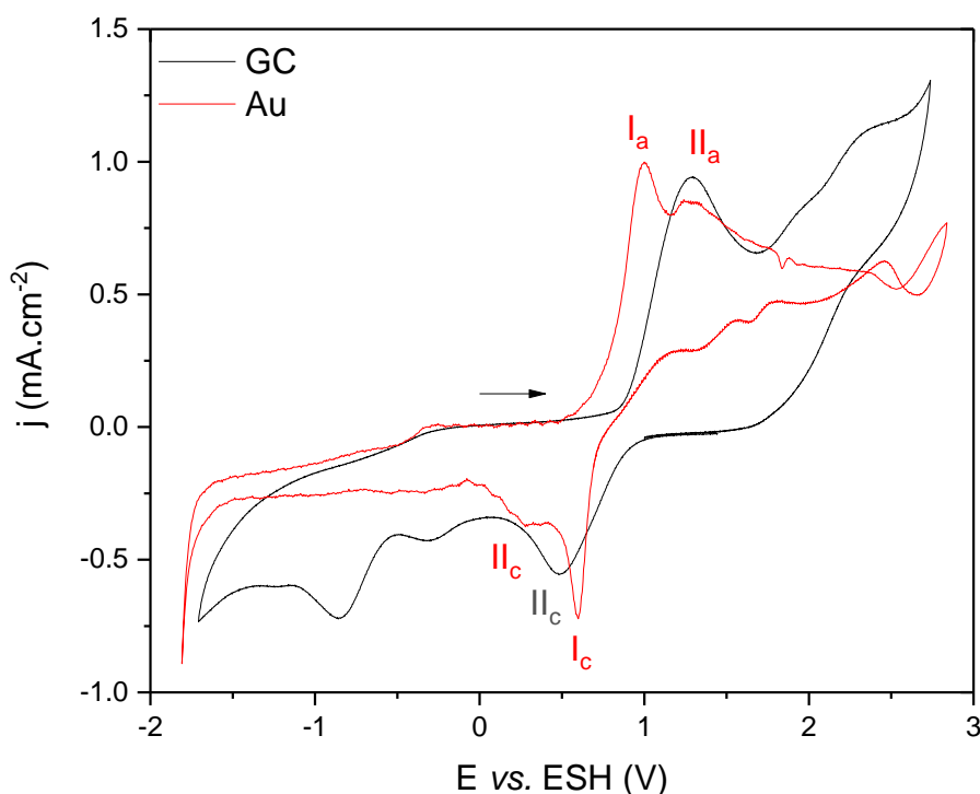
Figure II-37 - Voltampérogrammes cycliques à 50 \text{ mV.s}^{-1} obtenus sur des électrodes d'or (rouge) de carbone vitreux (noir) dans C_4C_1Im (NTf_2)_{0,97}(SCN)_{0,03} – T = 40 \text{ }^\circ\text{C}
