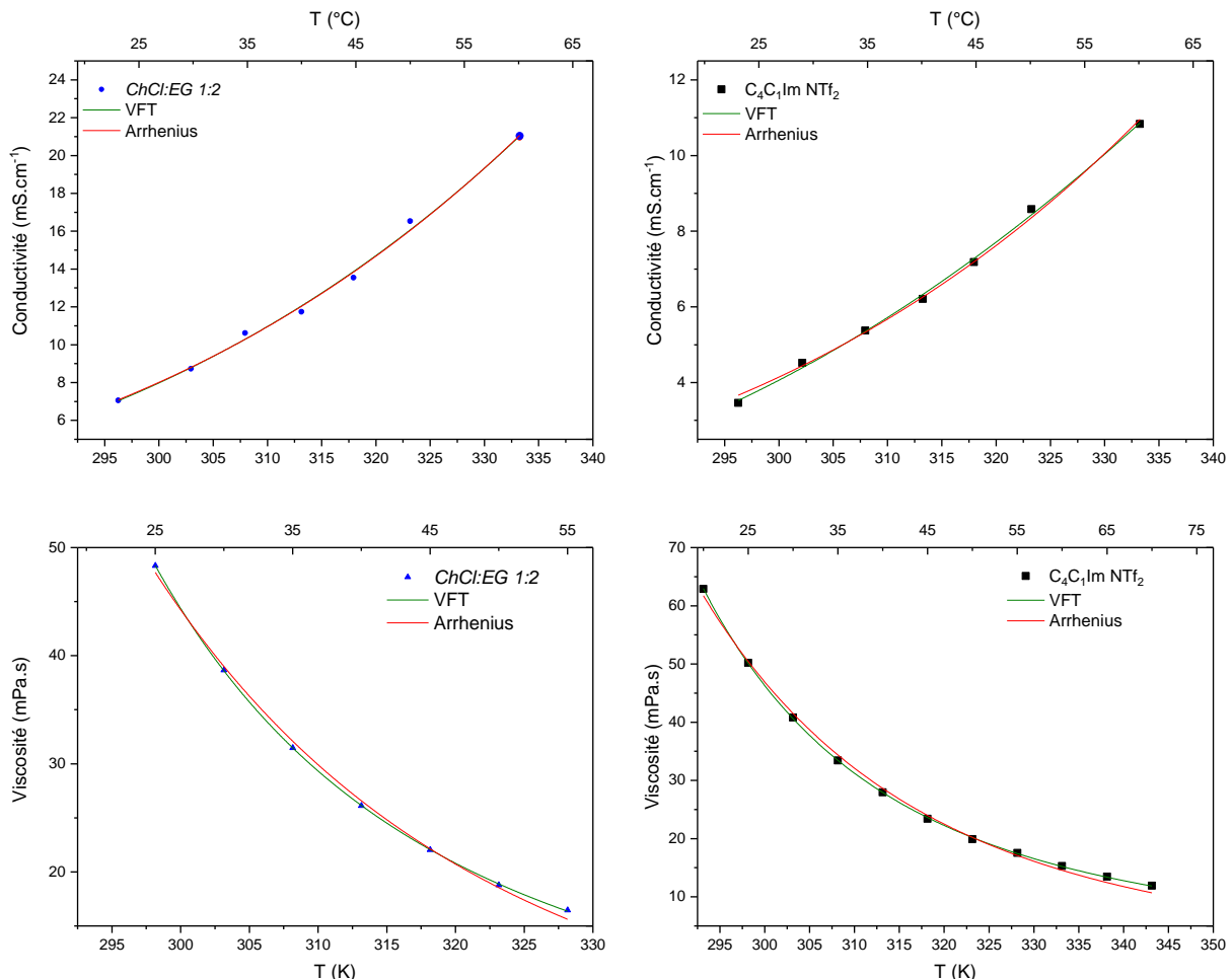
Figure III-17 - Meilleur ajustement des données pour l'équation VFT (vert) et d'Arrhenius (rouge) pour la conductivité ionique (haut gauche) et la viscosité (bas gauche) de ChCl:EG 1:2 et de la conductivité ionique (haut droite) et la viscosité (bas droite) de C 4 C 1 Im NTf 2
