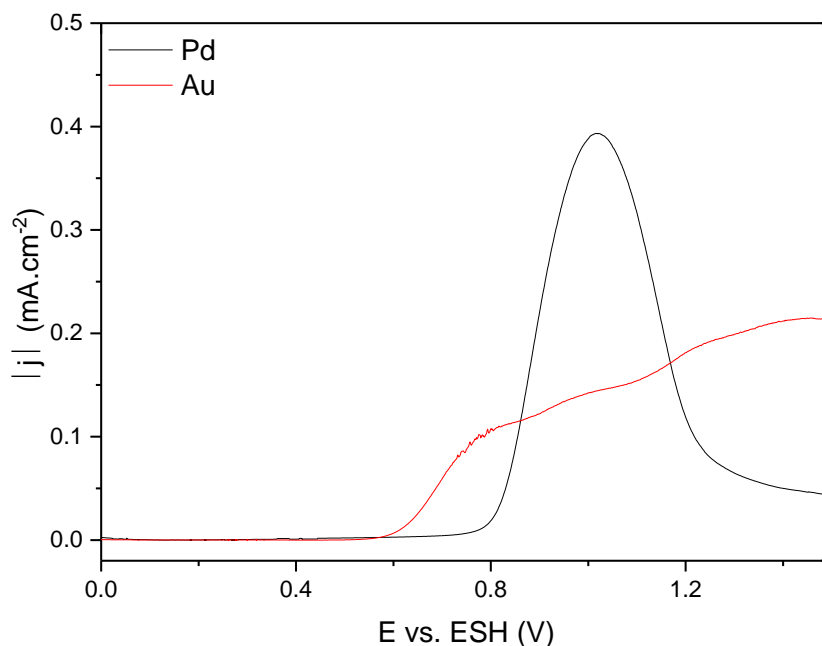
Figure II-16 - Voltampérogrammes linéaires à 0,167 \text{ mV}\cdot\text{s}^{-1} obtenus sur une électrode d'or (rouge) et de palladium (noir) dans C_4C_1Im (NTf_2)_{0,97}(SCN)_{0,03} - T = 40 \text{ }^\circ\text{C}
