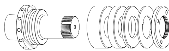
GWA HSK-E50 // \varnothing 31,75 mm ( 1\frac{1}{4} ) // RS \varnothing 60 mm
