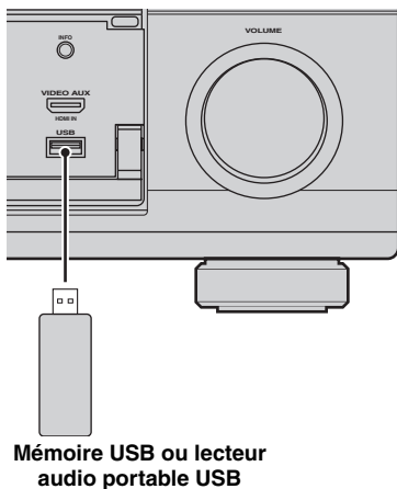
(Face avant)
