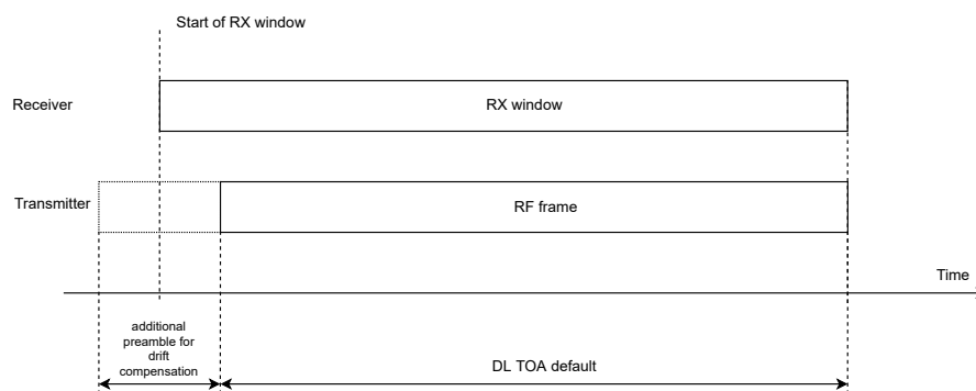
Fig. 5.44 Timedrift compensation
