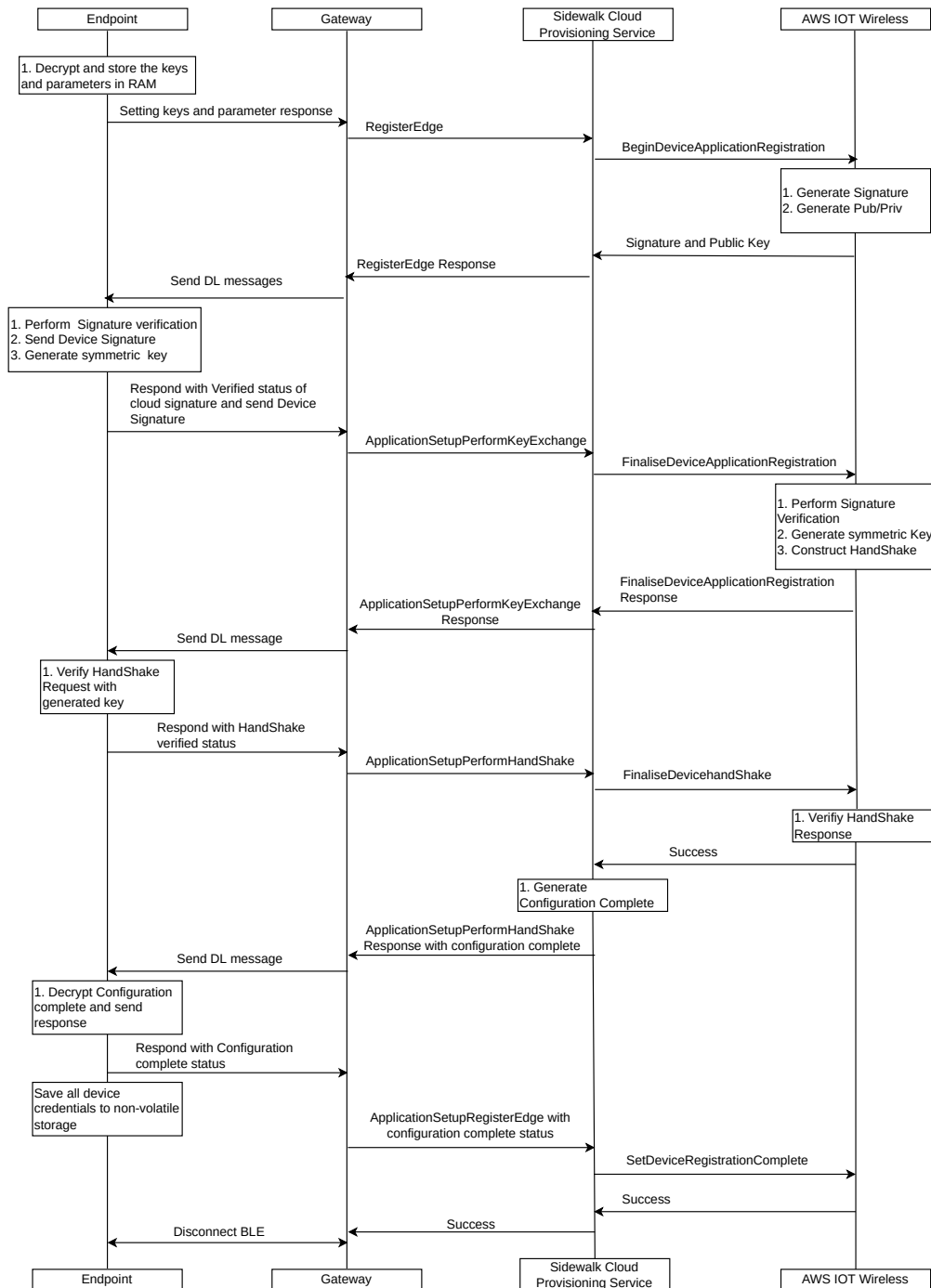
Fig. 6.21 BLE Endpoint registration 2of2
