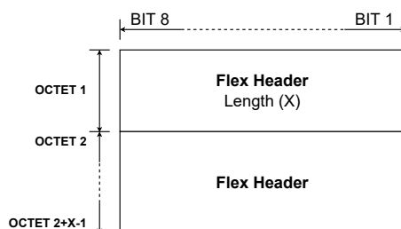
Fig. 6.12 BLE Data - Flex layer frame format
