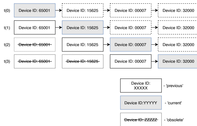
Fig. 4.11 ID rotation
