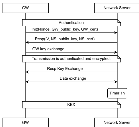
Fig. 4.10 TLS
