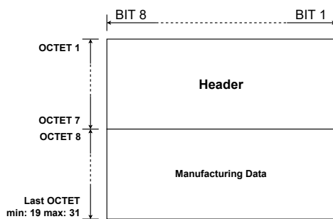
Fig. 6.3 BLE Beacon - Blocks
