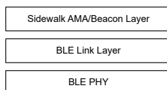
Fig. 6.1 BLE Beacon stack
