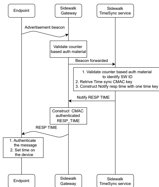
Fig. 6.22 BLE TimeSync flow
