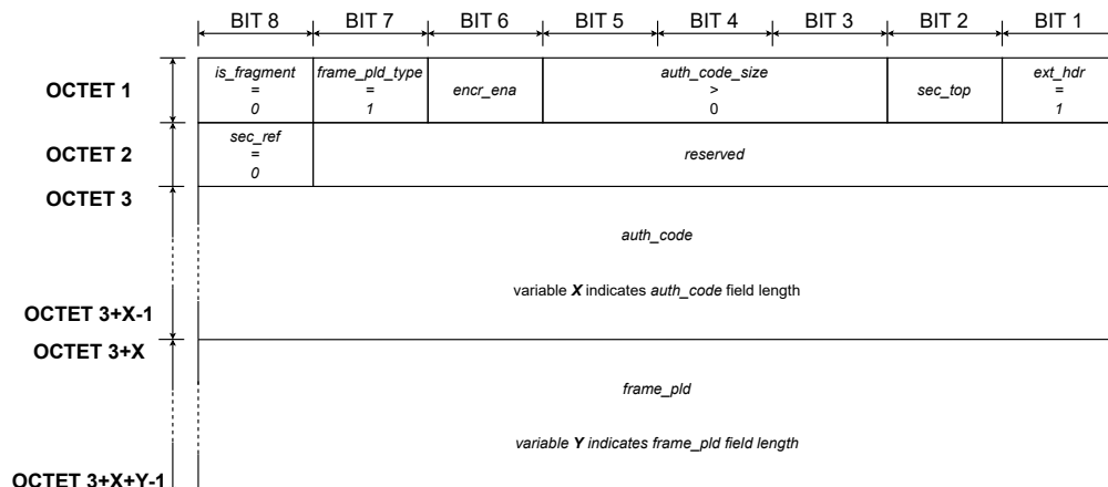
Fig. 5.22 Network layer - Frame format - Case 3A
