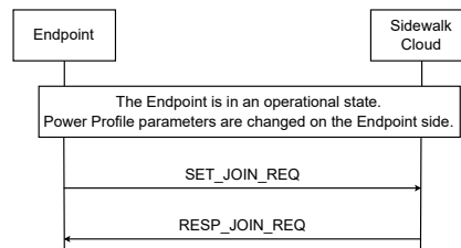
Fig. 7.5 Power profile parameter change
