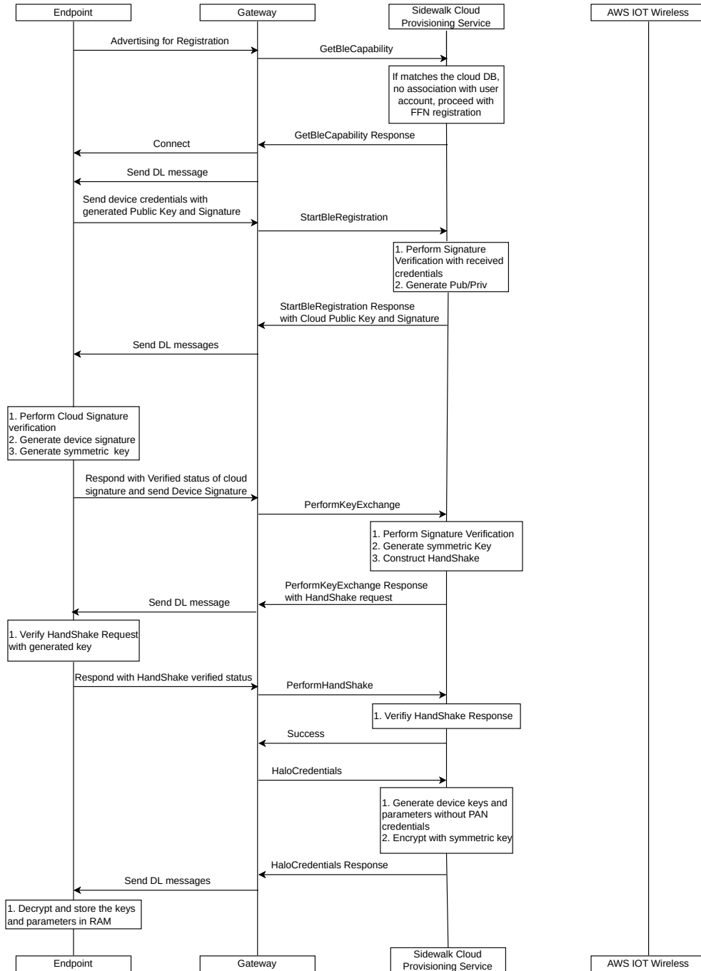
Fig. 6.20 BLE Endpoint registration 1 of 2
