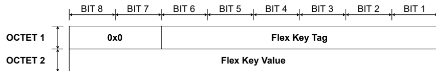
Fig. 6.16 Flex key coding - 1 byte optimized format
