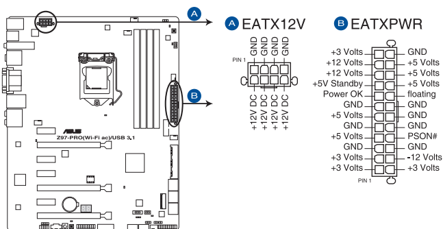
Connecteurs d'alimentation de la Z97-PRO (Wi-Fi ac) / USB 3.1
