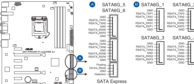
Connecteurs SATA 6.0Gbs de la Z97-PRO (Wi-Fi ac) / USB 3.1
