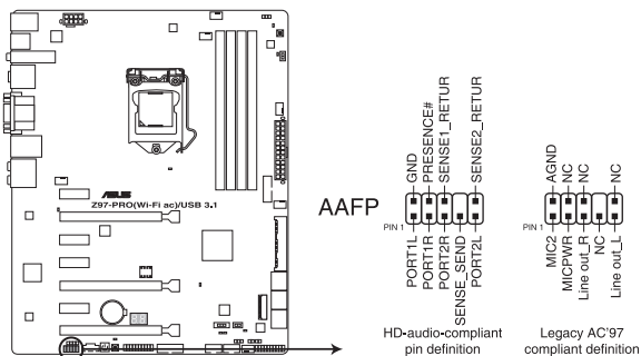
Connecteur audio pour panneau avant de la Z97-PRO (Wi-Fi ac) / USB 3.1
