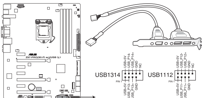
Connecteurs USB 2.0 de la Z97-PRO (Wi-Fi ac) / USB 3.1
