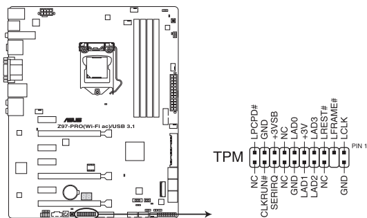
Connecteur TPM de la Z97-PRO (Wi-Fi ac) / USB 3.1
