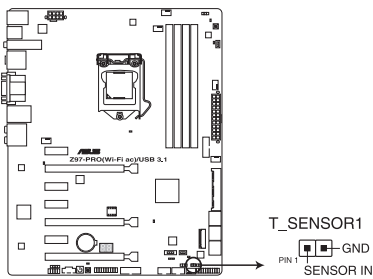
Connecteur pour câble à thermistance de la Z97-PRO (Wi-Fi ac) / USB 3.1
