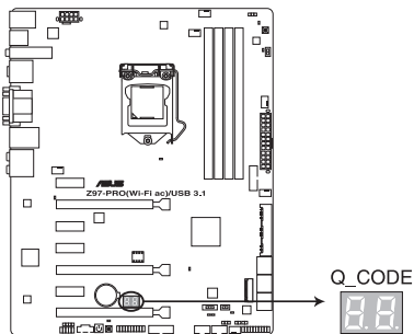
Témoins de débogage de la Z97-PRO (Wi-Fi ac) / USB 3.1
