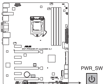
Bouton de mise sous tension de la Z97-PRO (Wi-Fi ac) / USB 3.1
