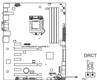
Connecteur DirectKey de la Z97-PRO (Wi-Fi ac) / USB 3.1
