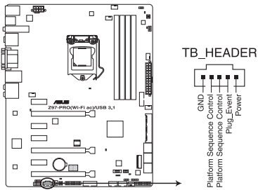
Connecteur Thunderbolt de la Z97-PRO (Wi-Fi ac) / USB 3.1
