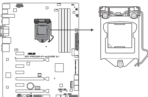
Interface de connexion LGA1150 de la Z97-PRO (Wi-Fi ac) / USB 3.1
