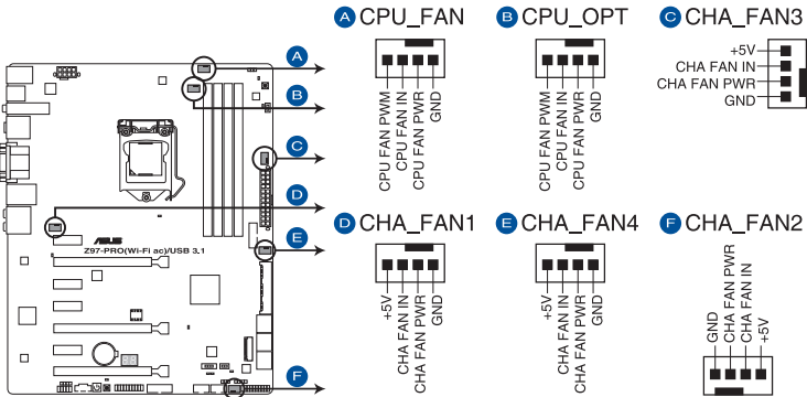
Connecteurs de ventilation de la Z97-PRO (Wi-Fi ac) / USB 3.1
