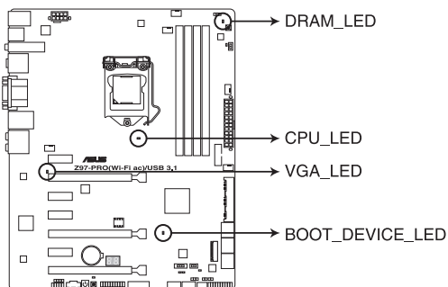
Témoins du POST de la Z97-PRO (Wi-Fi ac) / USB 3.1
