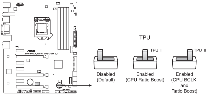
Interrupteur TPU de la Z97-PRO (Wi-Fi ac) / USB 3.1
