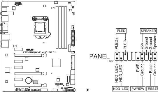
Connecteur panneau système de la Z97-PRO (Wi-Fi ac) / USB 3.1
