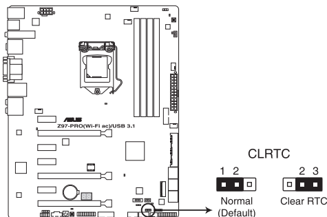
Jumper d'effacement de la mémoire CMOS de la Z97-PRO (Wi-Fi ac) / USB 3.1
