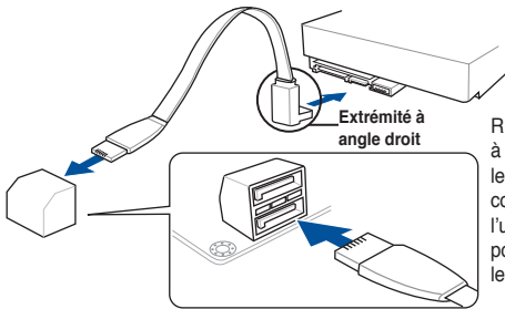
Connecteurs SATA 6.0Gbs de la Z97-PRO (Wi-Fi ac) / USB 3.1
