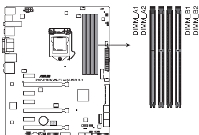
Interfaces de connexion pour modules mémoire DDR3 de la Z97-PRO (Wi-Fi ac) / USB 3.1
