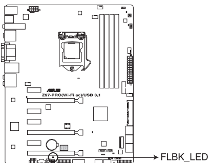
Témoin USB BIOS Flashback de la Z97-PRO (Wi-Fi ac) / USB 3.1
