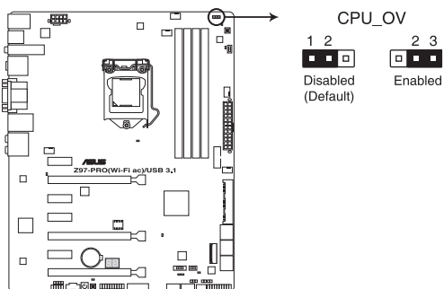
Jumper de surtension du processeur de la Z97-PRO (Wi-Fi ac) / USB 3.1
