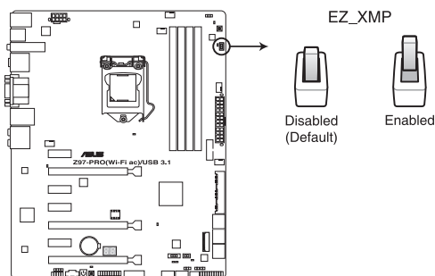
Interrupteur EZ XMP de la Z97-PRO (Wi-Fi ac) / USB 3.1
