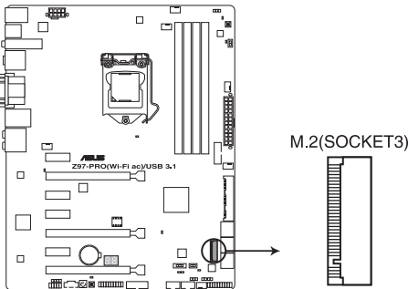
Connecteur M.2 de la Z97-PRO (Wi-Fi ac) / USB 3.1
