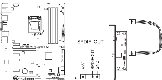
Connecteur audio numérique de la Z97-PRO (Wi-Fi ac) / USB 3.1
