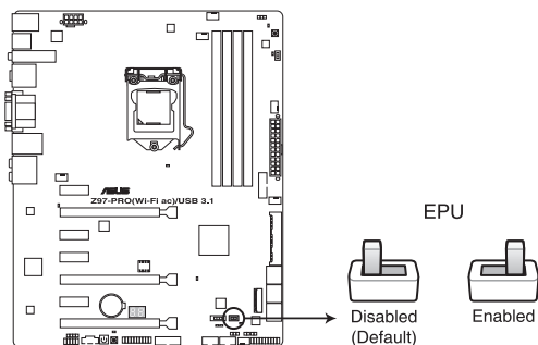
Interrupteur EPU de la Z97-PRO (Wi-Fi ac) / USB 3.1
