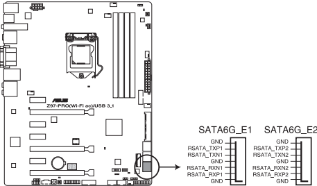
Connecteurs SATA 6Gb/s Marvell de la Z97-PRO (Wi-Fi ac) / USB 3.1
