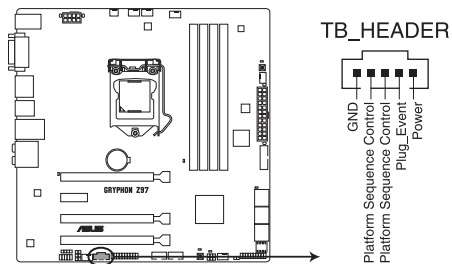
Connecteur Thunderbolt de la GRYPHON Z97
