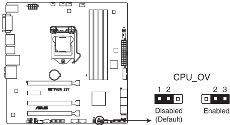
Jumper de surtension du processeur de la GRYPHON Z97
