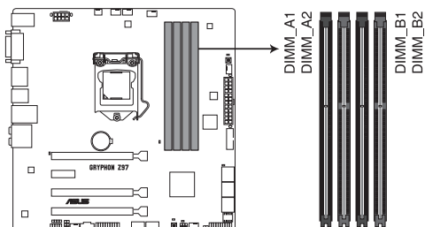
Interfaces de connexion pour modules mémoire DDR3 de la GRYPHON Z97
