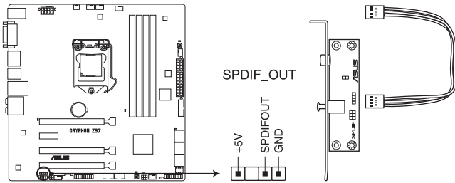
Connecteur audio numérique de la GRYPHON Z97
