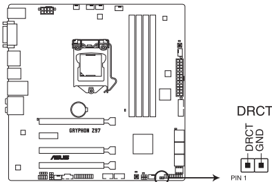
Connecteur DirectKey de la GRYPHON Z97
