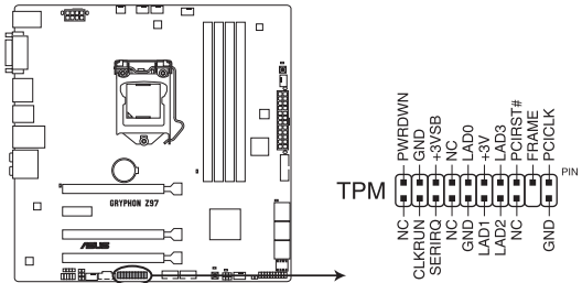
Connecteur TPM de la GRYPHON Z97
