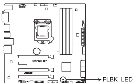
Témoin USB BIOS Flashback de la GRYPHON Z97
