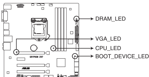
Témoins du POST de la GRYPHON Z97
