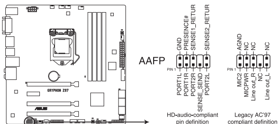
Connecteur audio pour panneau avant de la GRYPHON Z97
