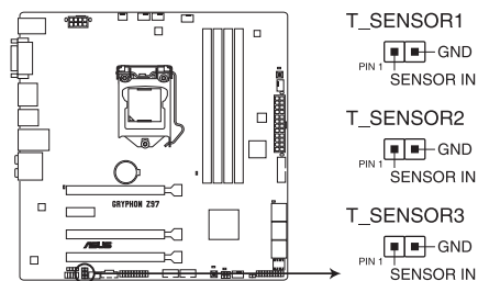
Connecteurs pour câbles à thermistance de la GRYPHON Z97
