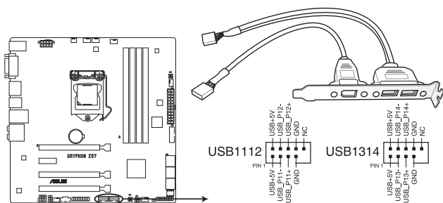
Connecteurs USB 2.0 de la GRYPHON Z97
