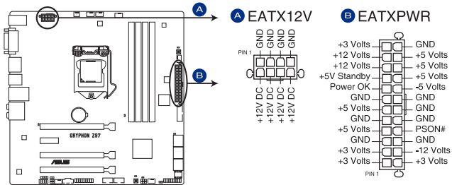
Connecteurs d'alimentation de la GRYPHON Z97
