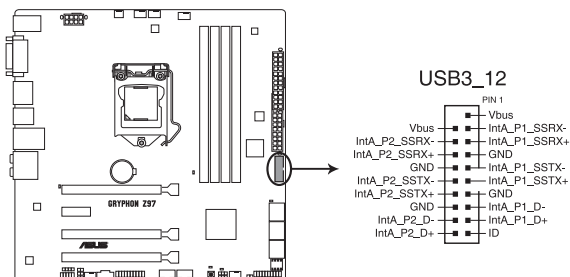
Connecteur USB 3.0 de la GRYPHON Z97
