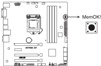
Bouton MemOK! de la GRYPHON Z97
