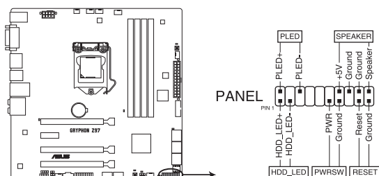
Connecteur panneau système de la GRYPHON Z97
