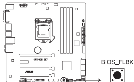
Bouton USB BIOS Flashback de la GRYPHON Z97
