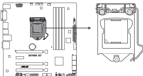
Interface de connexion LGA1150 de la GRYPHON Z97
