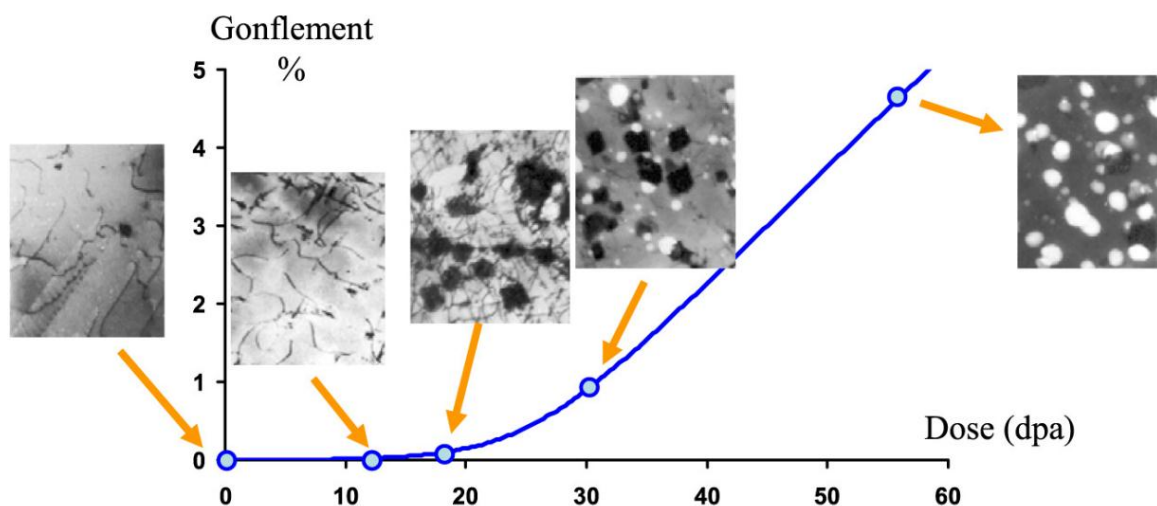
Figure 1.3 : Gonflement en fonction de la dose, pour un acier 316 hyperefflué irradié à 600°C, dans le réacteur à neutrons rapides PHENIX [Dubuisson (2011)].
