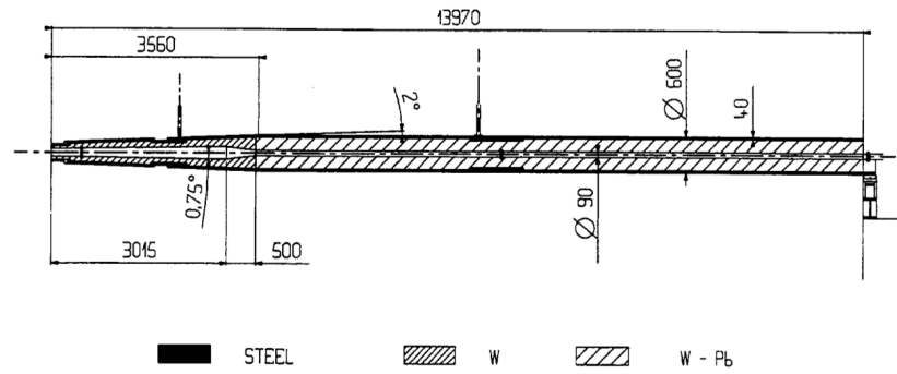
FIGURE 2.8 – Vue en coupe du blindage du tube faisceau au niveau du spectromètre à muons du détecteur ALICE.
