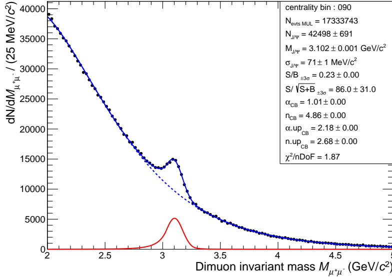
FIGURE 4.6 – Spectre brut de masse invariante des dimuons intégrés en p_T , y et centralité. Les résultats de l’ajustement pour l’intervalle en masse 2 < M_{\mu^+\mu^-} < 5 \text{ GeV}/c^2 sont reportés dans la légende.
