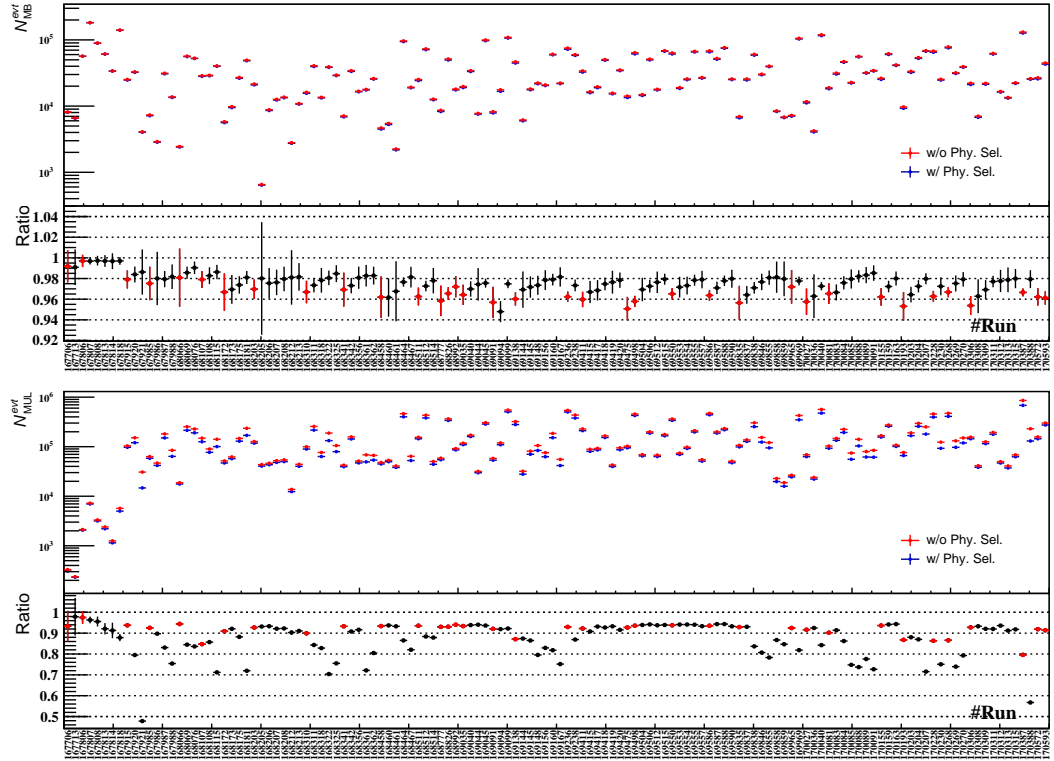
FIGURE 6.4 – Distributions des nombres d'événements par run avant et après application de la physics selection et du rapport associé pour la classe de déclenchement MB (haut) et MUL (bas). Les points rouges du rapport correspondent aux premiers runs des remplissages du LHC.
