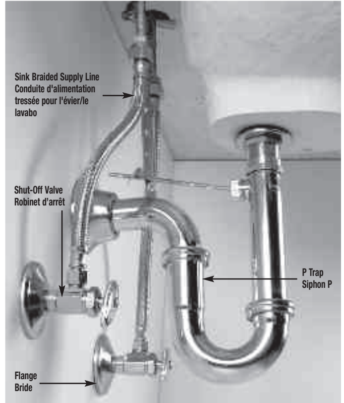
Sink Water Supply Hook Up / Raccord de l'alimentation en eau de l'évier
