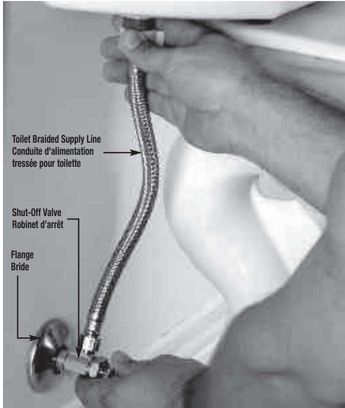
Toilet Water Supply Hook Up / Raccord de l'alimentation en eau de la toilette
