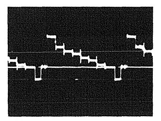
① 1.0Vp-p (H)
