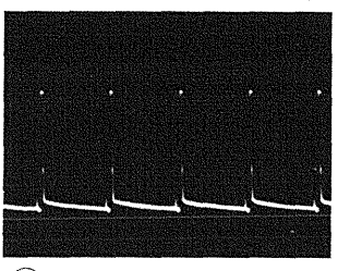
⑥ 12Vp-p (H)
