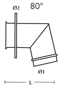
Art. nr PS11661 80° Ø 60 mm
