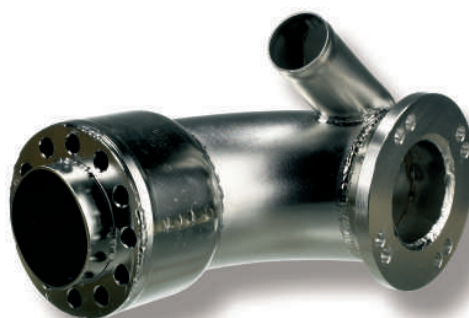
Art. nr 16810 (Yanmar 6 YL Serie)
