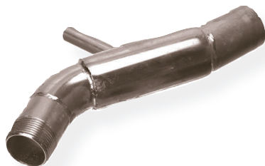
Art. nr 16100 (Volvo MD 1-3, 6, 7, 11, 17) ex. fläns / excl. flange
