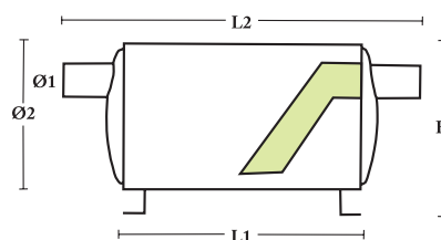
Typ A / Type A Rak anslutning in/ut Straight in/out
