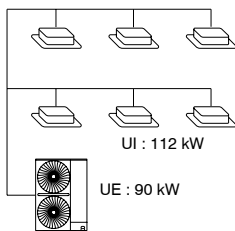
Système VRF traditionnel
