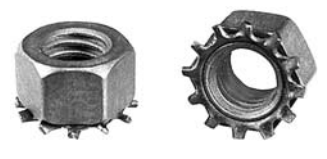
3/8-16 9/16 AF .66 OD .39 OAH PY, 34663-S, 271191
