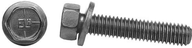
3/8-16 x 1 7/8 9/16 AF .75 CONICAL LCO, 6027876
