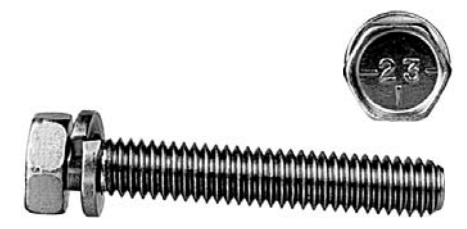
5/16-18 x 2.0 1/2 AF .55 SPLIT KFH, 376396-S
