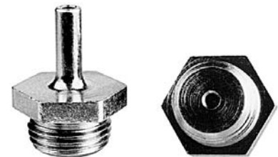
5/8-18 x 3/16 HOSE 3/4 AF 1.07 OAL KKC, C7AF-12A022-A
