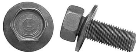
3/8-24 x 1.0 9/16 AF .88 CONICAL KYT
