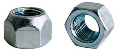
1/2-20 RH 3/4 AF .56 OAH KNB, 2409826 ♣
