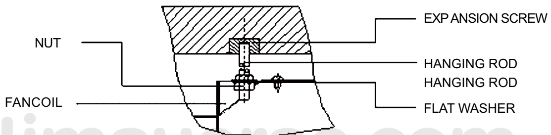
Fig.3 DETAIL A:
