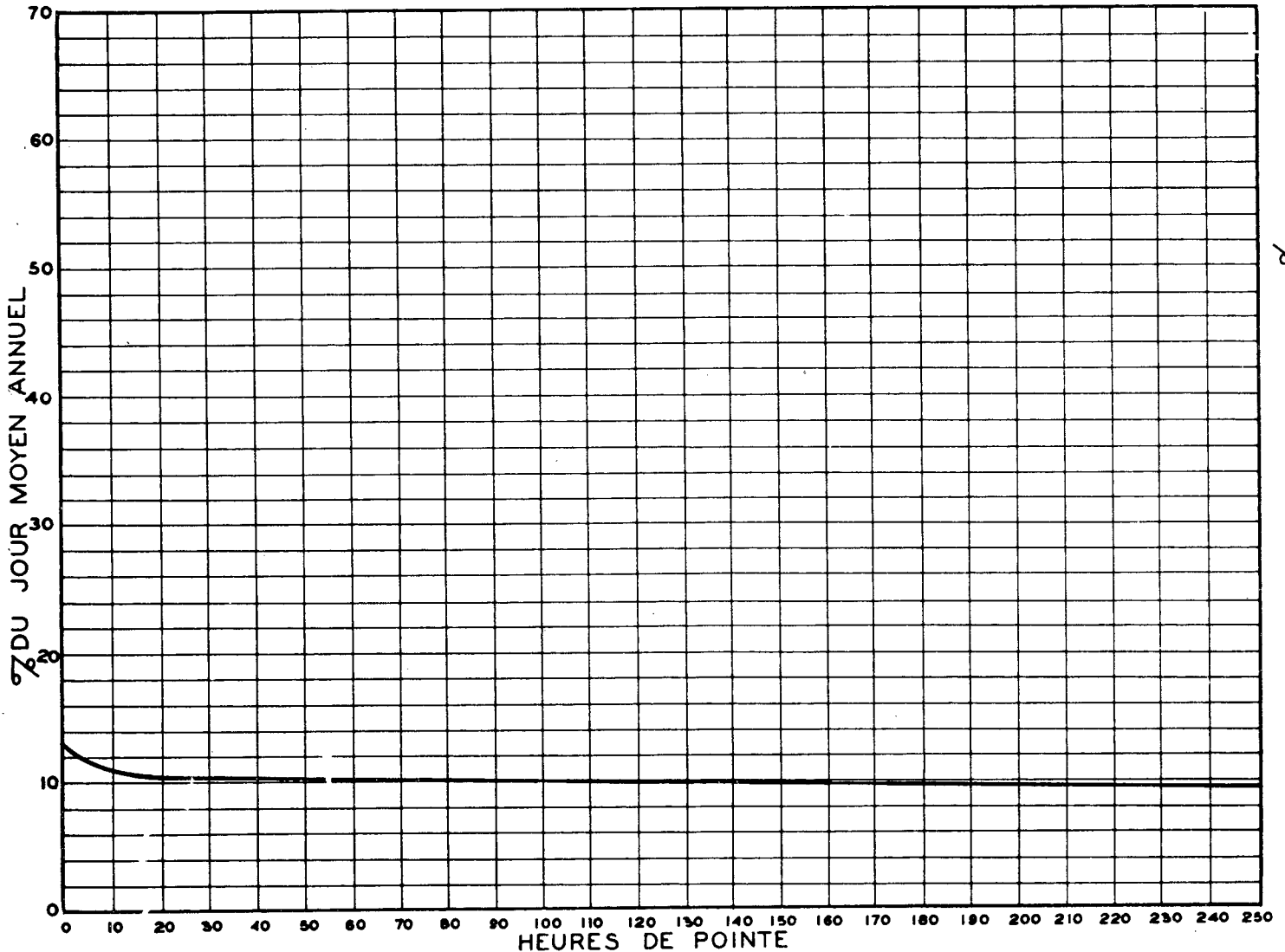
RELATION ENTRE LES HEURES DE POINTE ET LE JOUR MOYEN ANNUEL STATION: PONT TUNNEL LAFONTAINE VOIE NORD ROUTE N° 20-62-602
