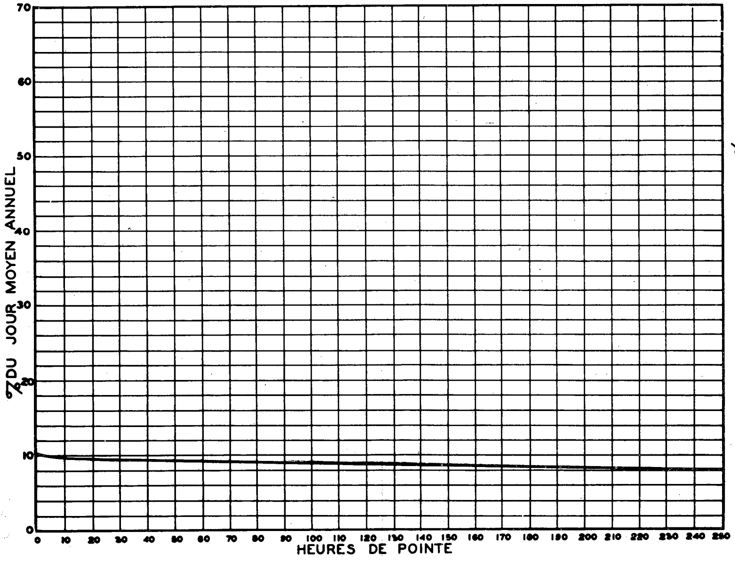
RELATION ENTRE LES HEURES DE POINTE ET LE JOUR MOYEN ANNUEL STATION: PONT MERCIER 2VOIES ROUTE N° 4-63-83
