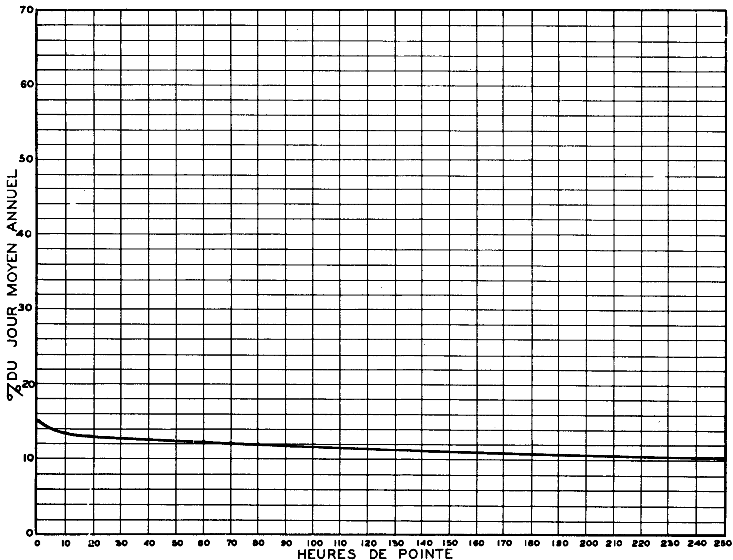
RELATION ENTRE LES HEURES DE POINTE ET LE JOUR MOYEN ANNUEL STATION: POINTE DU LAC ROUTE N° 2-4-54
