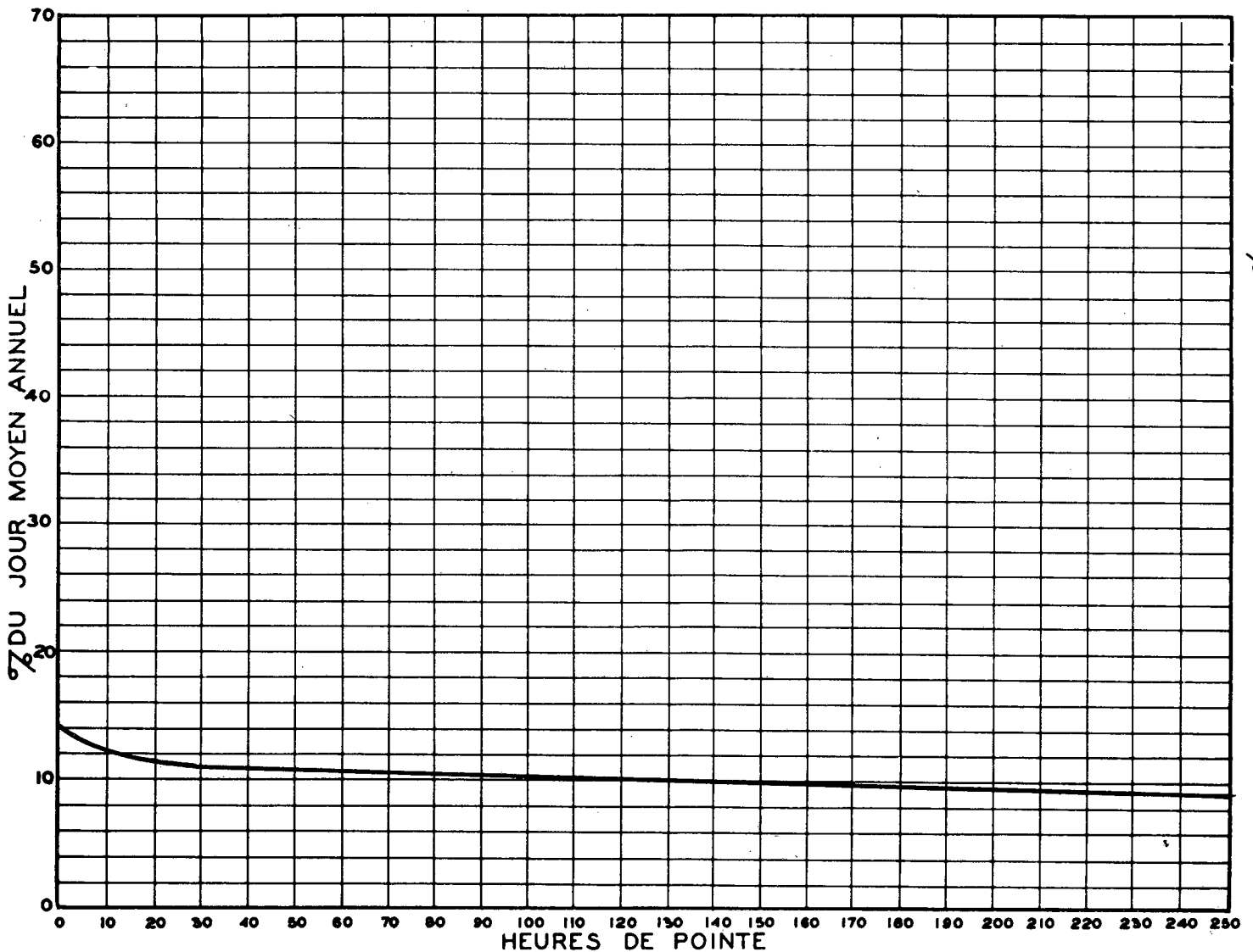
RELATION ENTRE LES HEURES DE POINTE ET LE JOUR MOYEN ANNUEL STATION: DOUVILLE ROUTE N° 9-61-65
