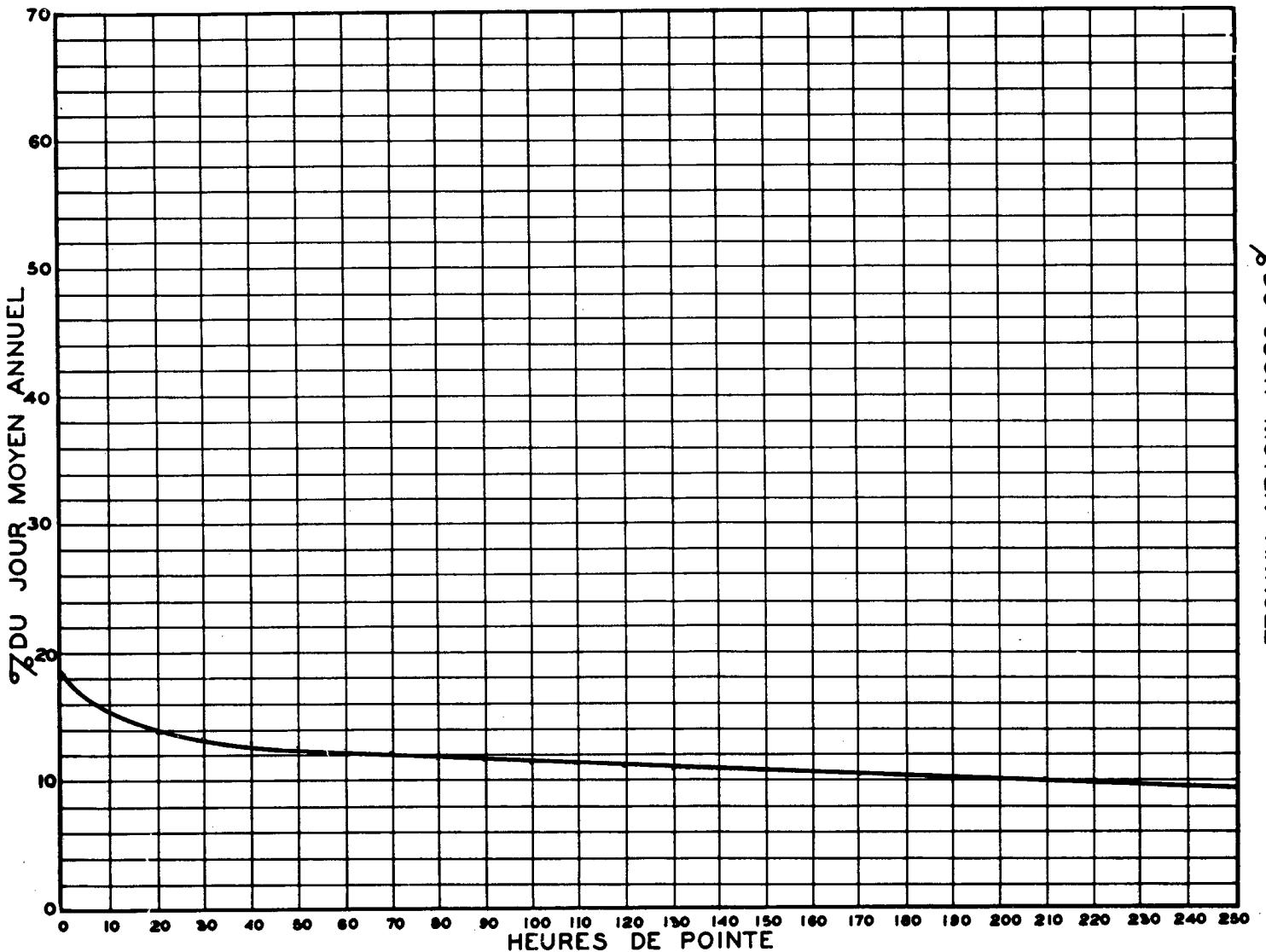
RELATION ENTRE LES HEURES DE POINTE ET LE JOUR MOYEN ANNUEL STATION: MERCIER ROUTE N° 4-62-61
