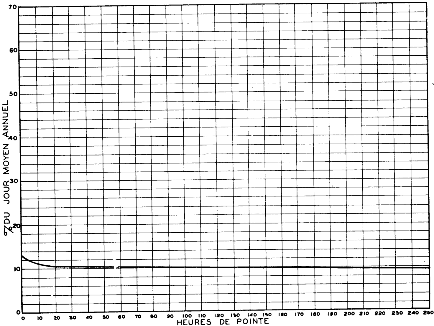
RELATION ENTRE LES HEURES DE POINTE ET LE JOUR MOYEN ANNUEL STATION: PONT TUNNEL LAFONTAINE 2 VOIES ROUTE N° 20-62-602
