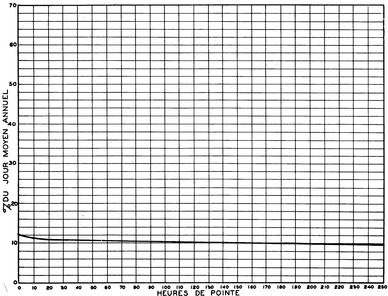
RELATION ENTRE LES HEURES DE POINTE ET LE JOUR MOYEN ANNUEL — STATION: HULL ROUTE N° 11-7-71
