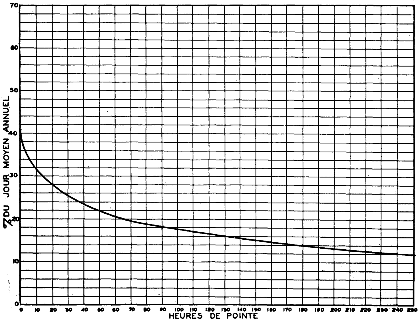
RELATION ENTRE LES HEURES DE POINTE ET LE JOUR MOYEN ANNUEL STATION: CHARLESBOURG VOIE OUEST ROUTE N° 54-31-1
