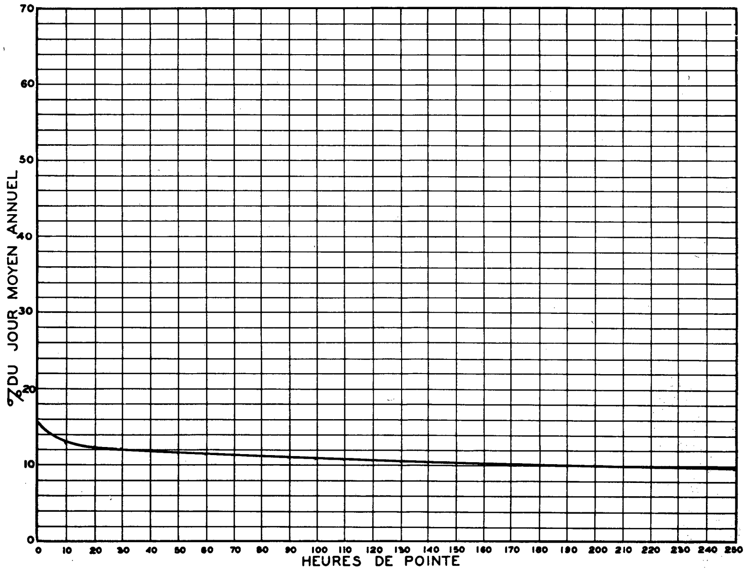
RELATION ENTRE LES HEURES DE POINTE ET LE JOUR MOYEN ANNUEL STATION: WINDSOR ROUTE N° 5-5-10
