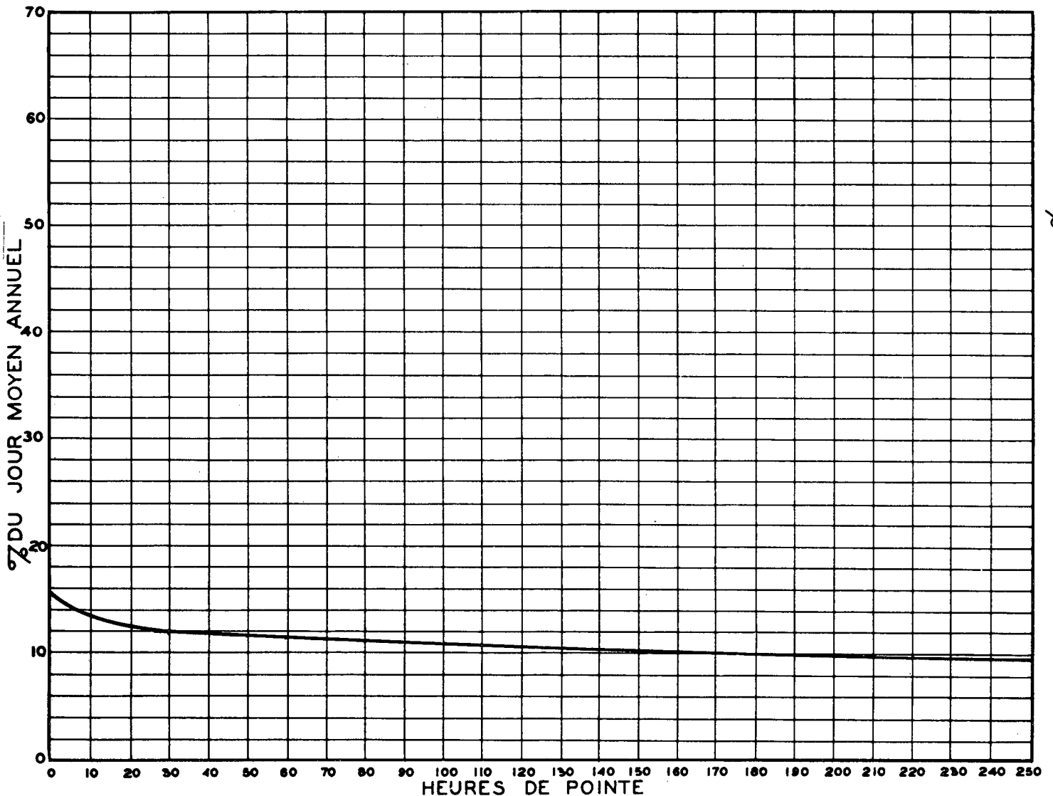
RELATION ENTRE LES HEURES DE POINTE ET LE JOUR MOYEN ANNUEL STATION: MAGOG 2 VOIES ROUTE N° 1-5-3
