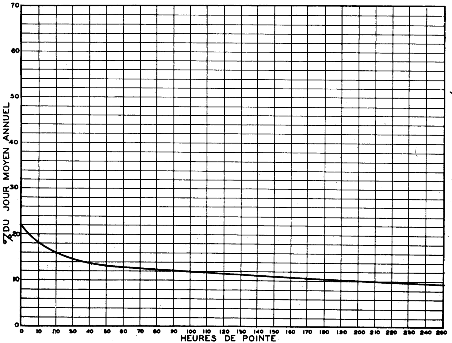
RELATION ENTRE LES HEURES DE POINTE ET LE JOUR MOYEN ANNUEL STATION: CHARLESBOURG 2 VOIES ROUTE N° 54-31-1
