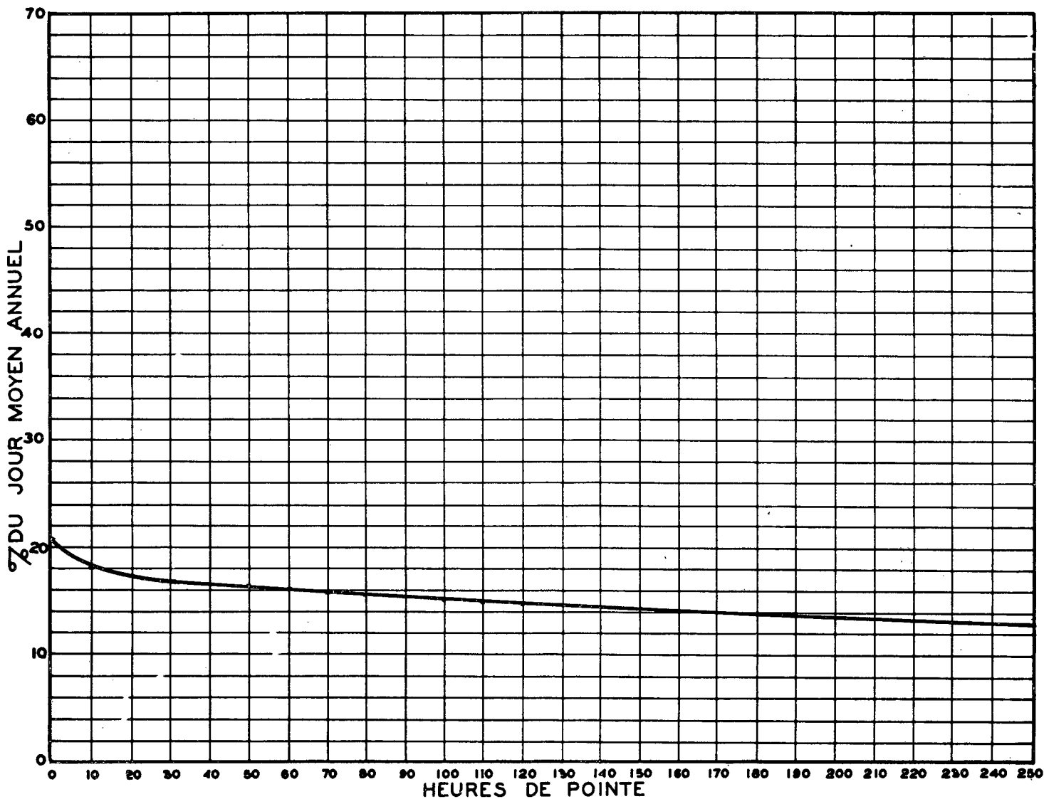
RELATION ENTRE LES HEURES DE POINTE ET LE JOUR MOYEN ANNUEL STATION: POINTE-FORTUNE ROUTE N° 40-63-980
