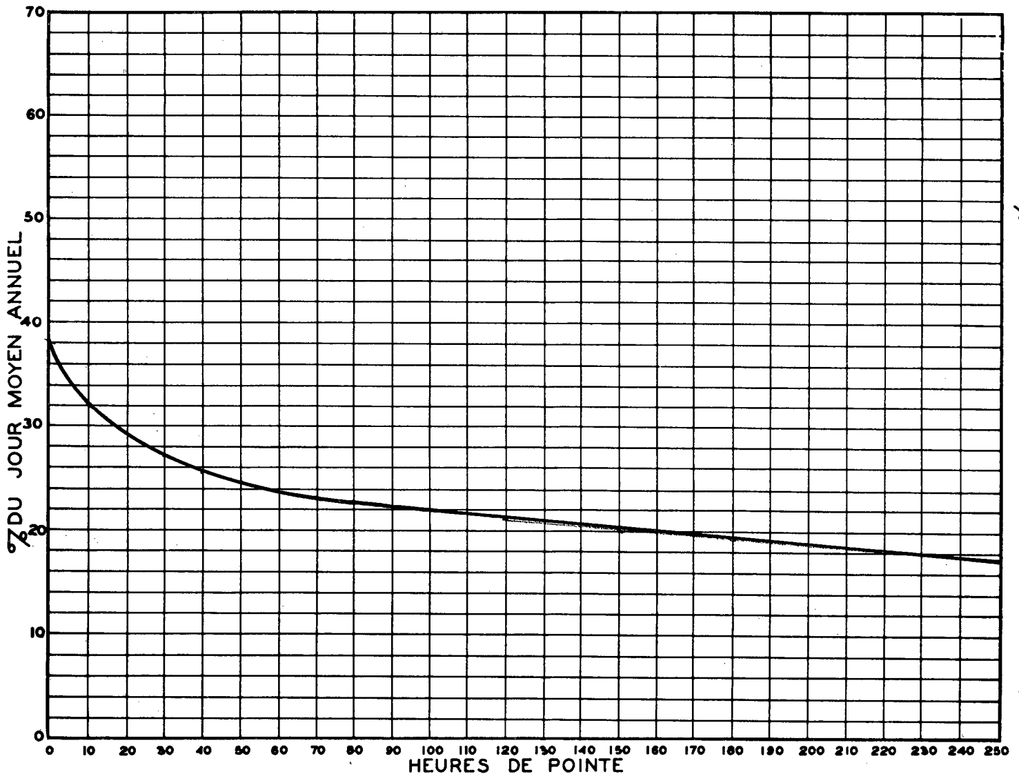
RELATION ENTRE LES HEURES DE POINTE ET LE JOUR MOYEN ANNUEL STATION: ST-JEAN-BOSCO ROUTE N° 19-4-4
