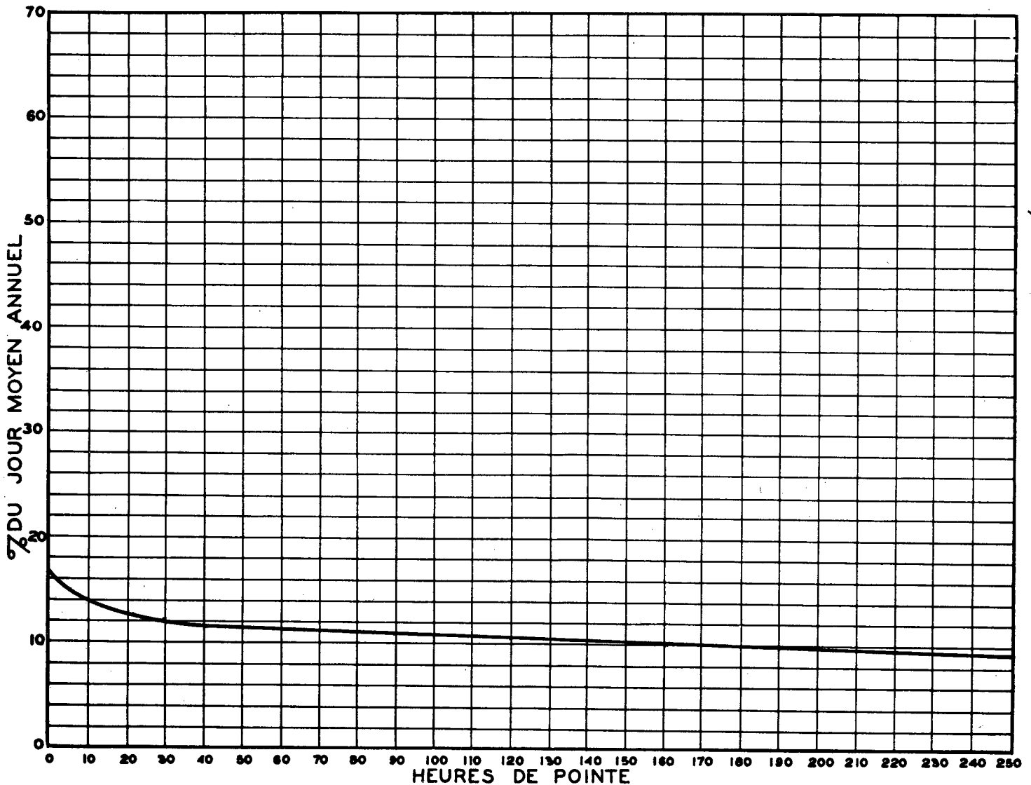
RELATION ENTRE LES HEURES DE POINTE ET LE JOUR MOYEN ANNUEL — STATION: ST-NICOLAS VOIE EST — — — — — ROUTE N° RS-32-199 — — — — —
