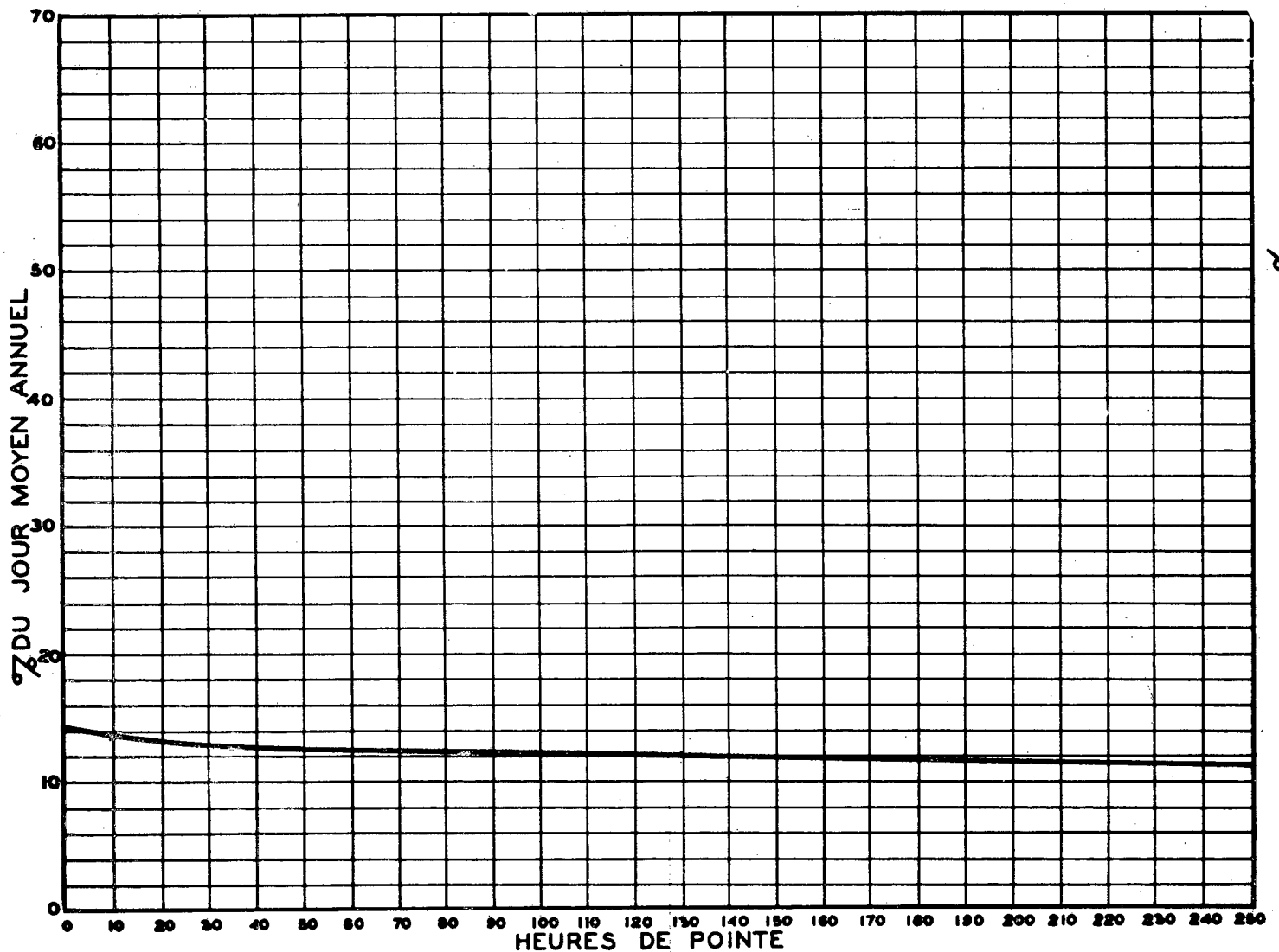
RELATION ENTRE LES HEURES DE POINTE ET LE JOUR MOYEN ANNUEL — STATION: DORVAL VOIE SUD ROUTE N° 20-63-752
