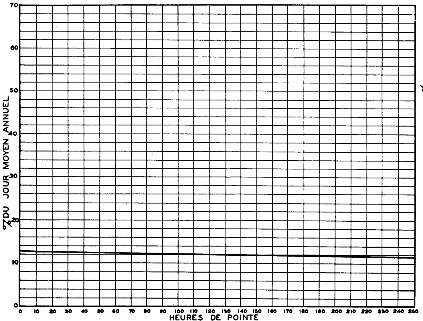
RELATION ENTRE LES HEURES DE POINTE ET LE JOUR MOYEN ANNUEL STATION: LAVAL VOIE EST ROUTE N° 11-63-80
