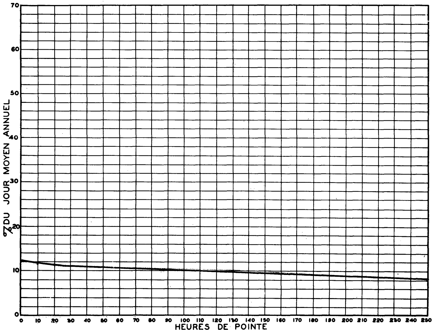
RELATION ENTRE LES HEURES DE POINTE ET LE JOUR MOYEN ANNUEL STATION: ST-HUBERT ROUTE N° 9-62-68
