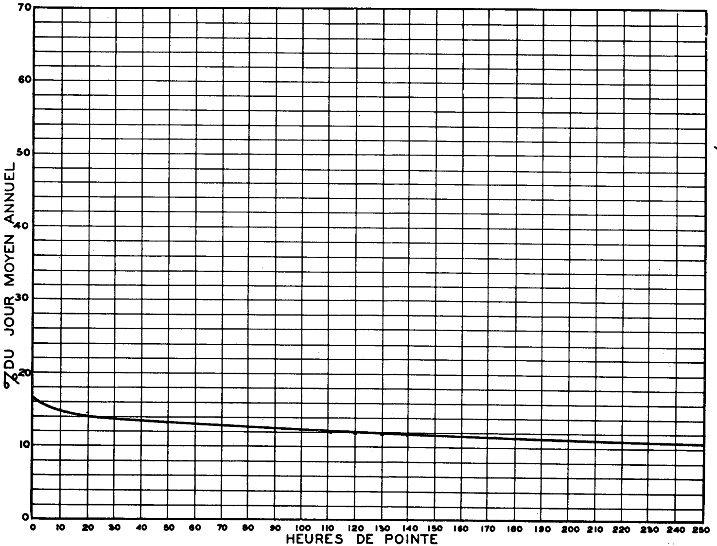
RELATION ENTRE LES HEURES DE POINTE ET LE JOUR MOYEN ANNUEL STATION: AMOUI ROUTE N° 6-1-3
