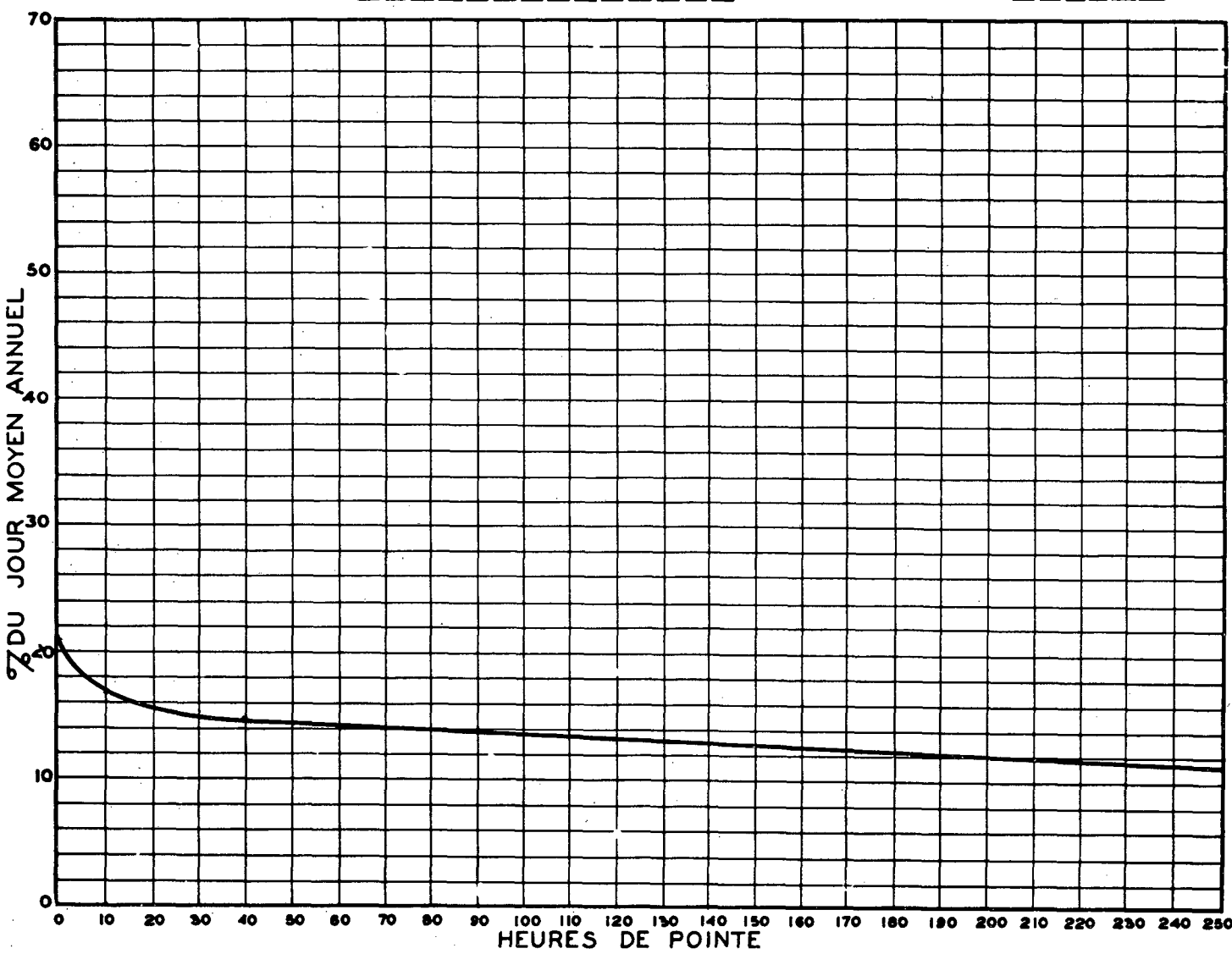
RELATION ENTRE LES HEURES DE POINTE ET LE JOUR MOYEN ANNUEL — STATION: ST-PIERRE-D'ESCOURT ROUTE N° 51-1-2
