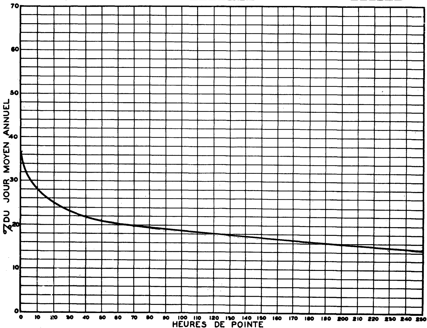
RELATION ENTRE LES HEURES DE POINTE ET LE JOUR MOYEN ANNUEL STATION: ST-MATHIEU-DE-DIXVILLE ROUTE N° 22-5-4
