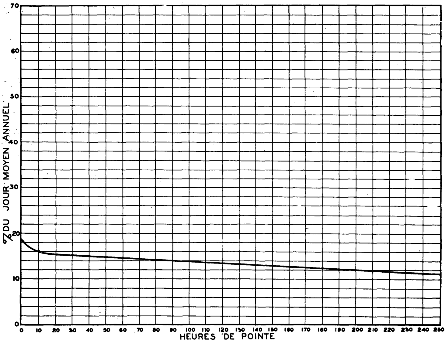
RELATION ENTRE LES HEURES DE POINTE ET LE JOUR MOYEN ANNUEL STATION: ST-LEONARD ROUTE N° 13-4-13
