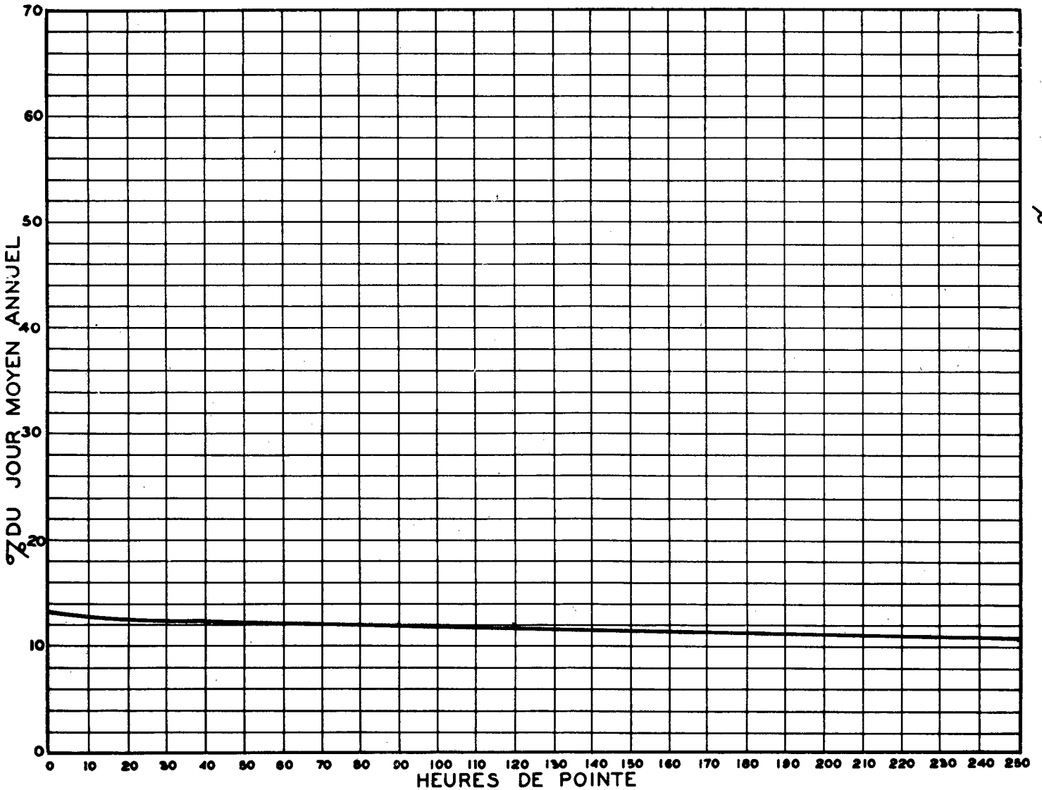
RELATION ENTRE LES HEURES DE POINTE ET LE JOUR MOYEN ANNUEL STATION: LAVAL VOIE OUEST ROUTE N° 11-63-80
