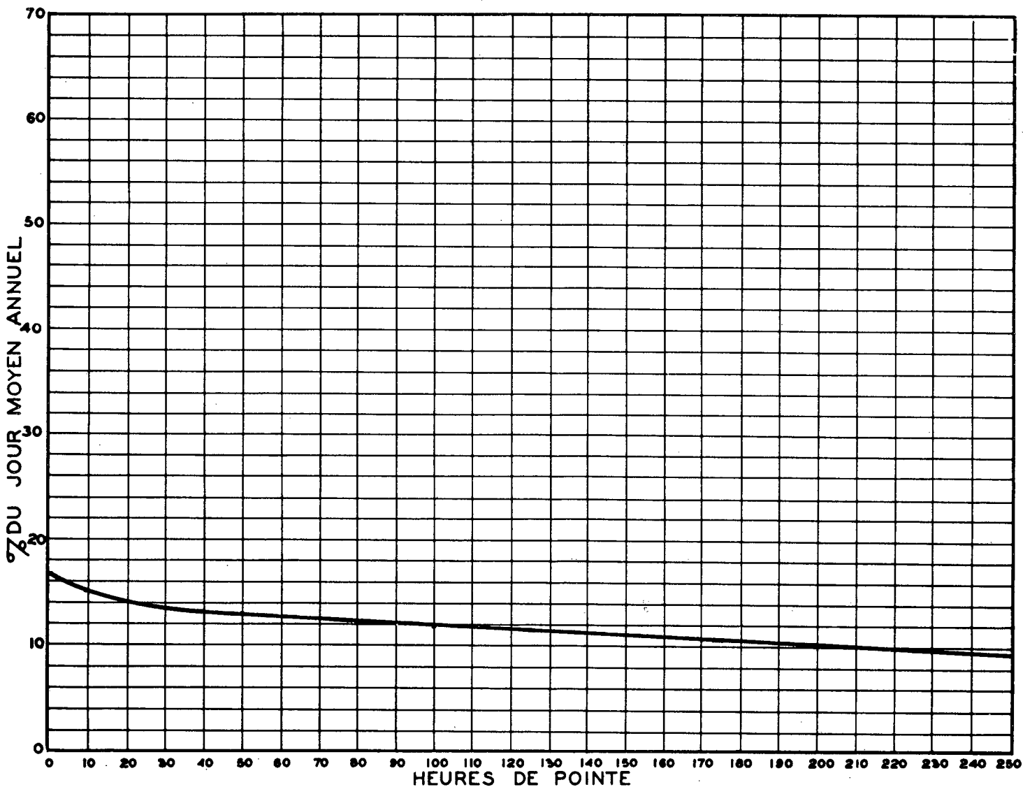
RELATION ENTRE LES HEURES DE POINTE ET LE JOUR MOYEN ANNUEL STATION: ST-JANVIER ROUTE N° 11-63-63
