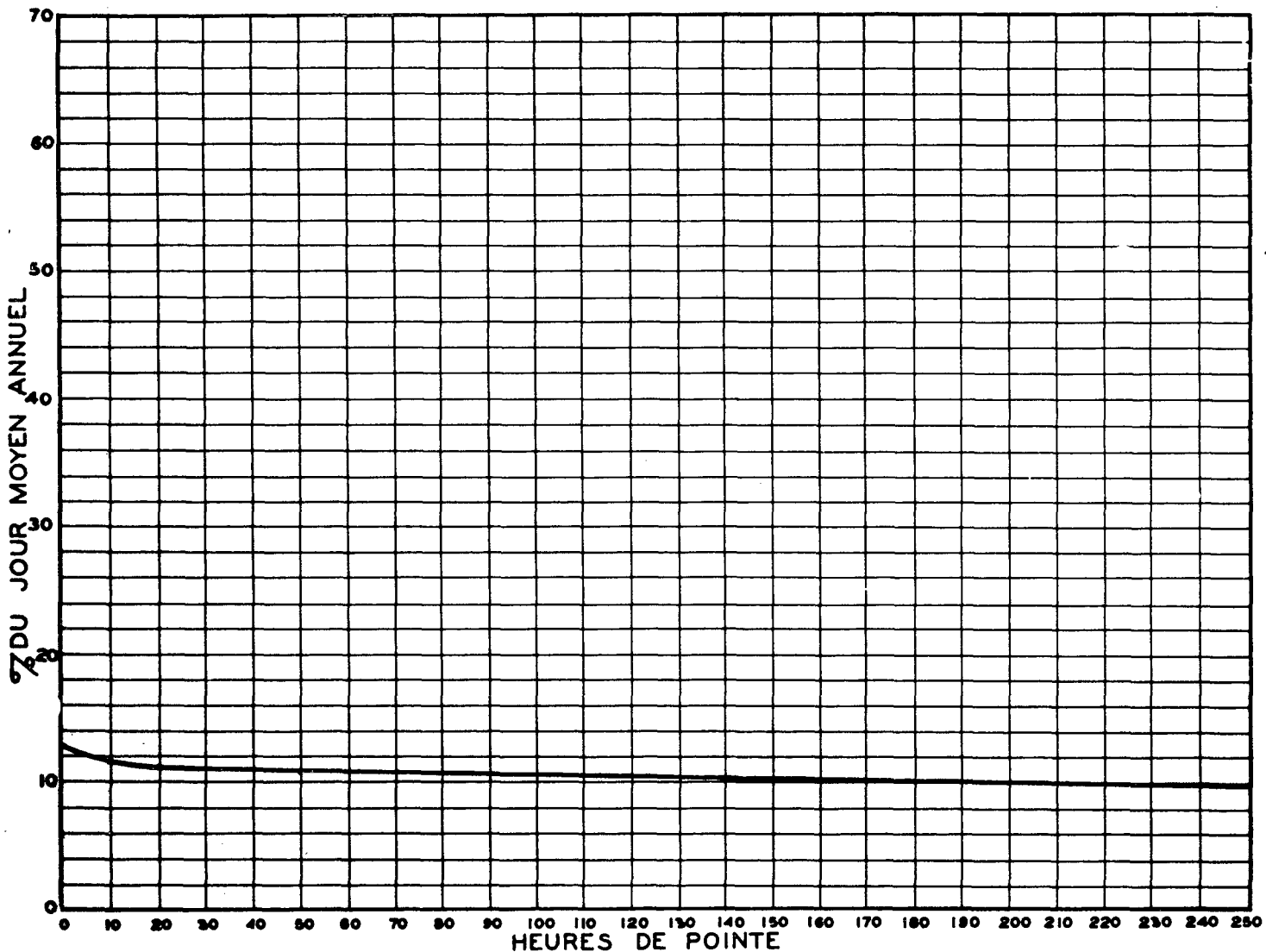
RELATION ENTRE LES HEURES DE POINTE ET LE JOUR MOYEN ANNUEL — STATION: PONT TUNEL LAFONTAINE VOIE SUD ROUTE N° 20-62-602
