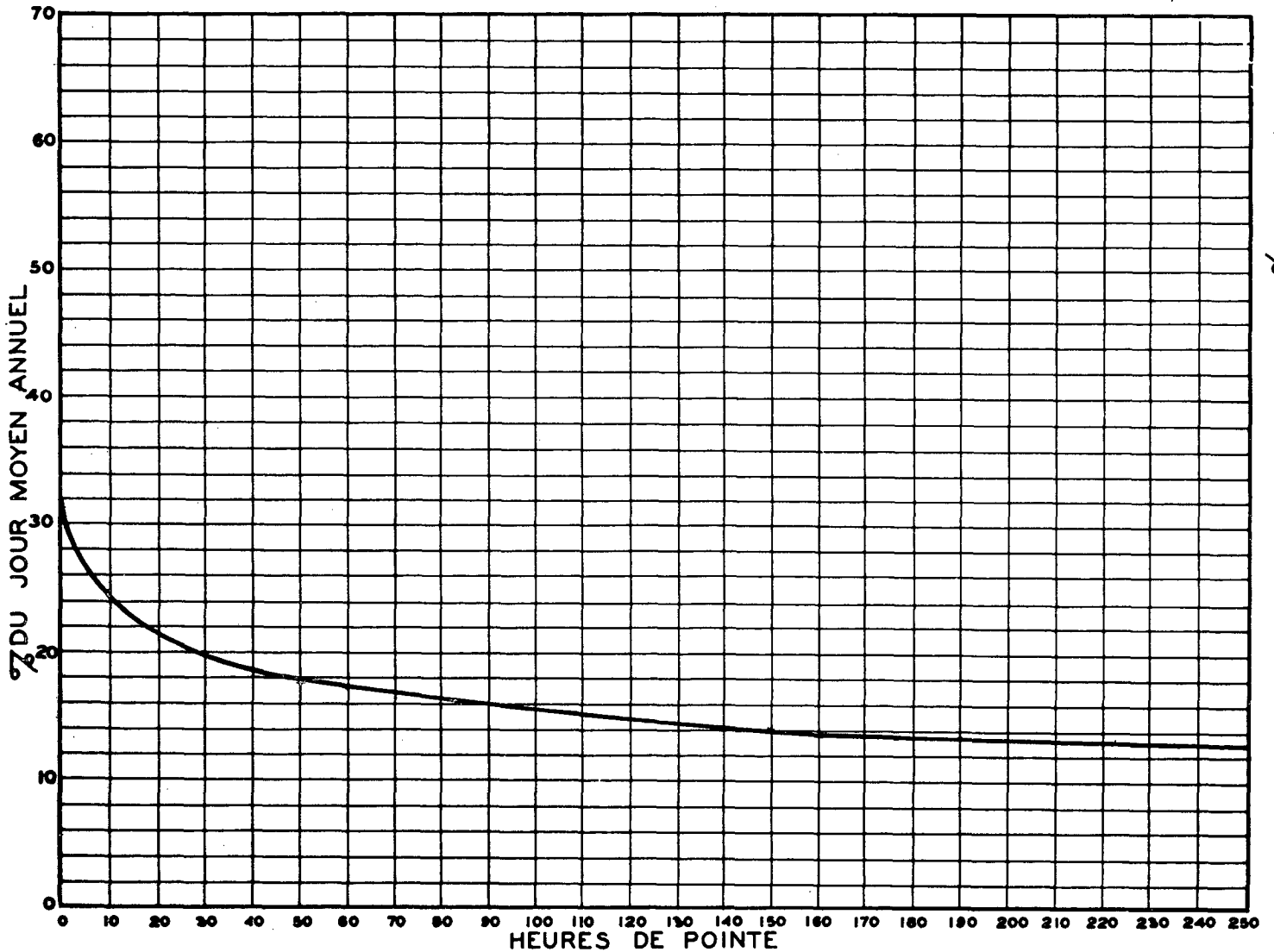
RELATION ENTRE LES HEURES DE POINTE ET LE JOUR MOYEN ANNUEL — STATION: VILLEROY VOIE NORD ROUTE N° 20-32-372
