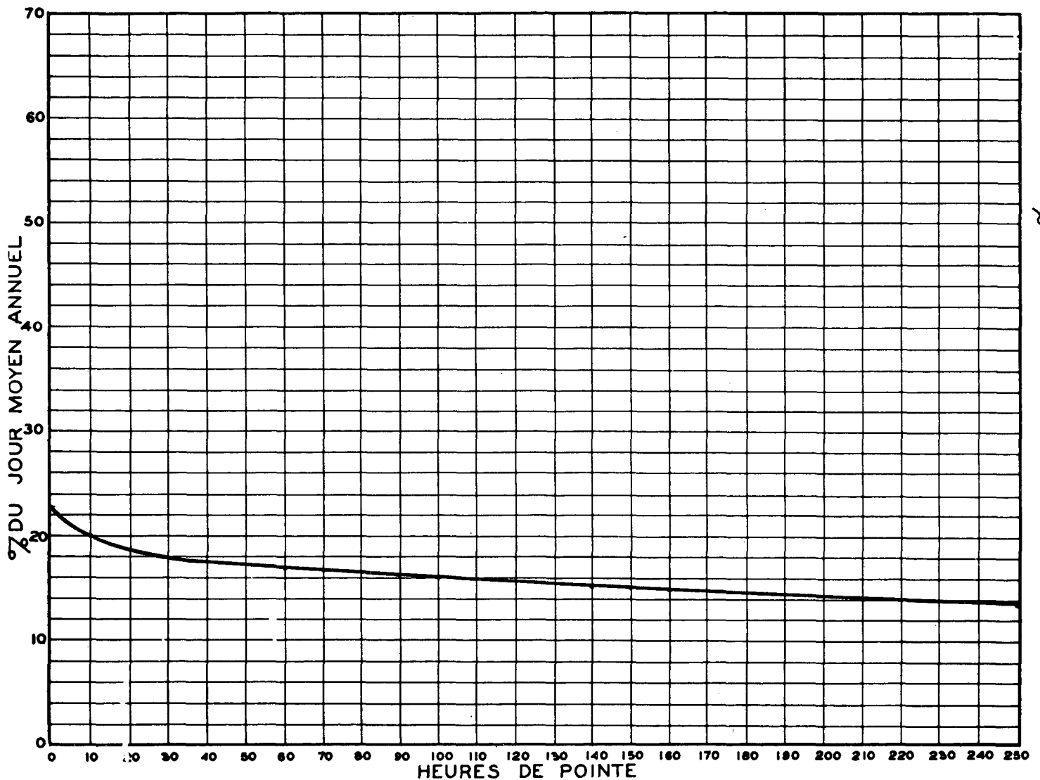
RELATION ENTRE LES HEURES DE POINTE ET LE JOUR MOYEN ANNUEL — STATION: ST-MATHIEU ROUTE N° 15-62-900
