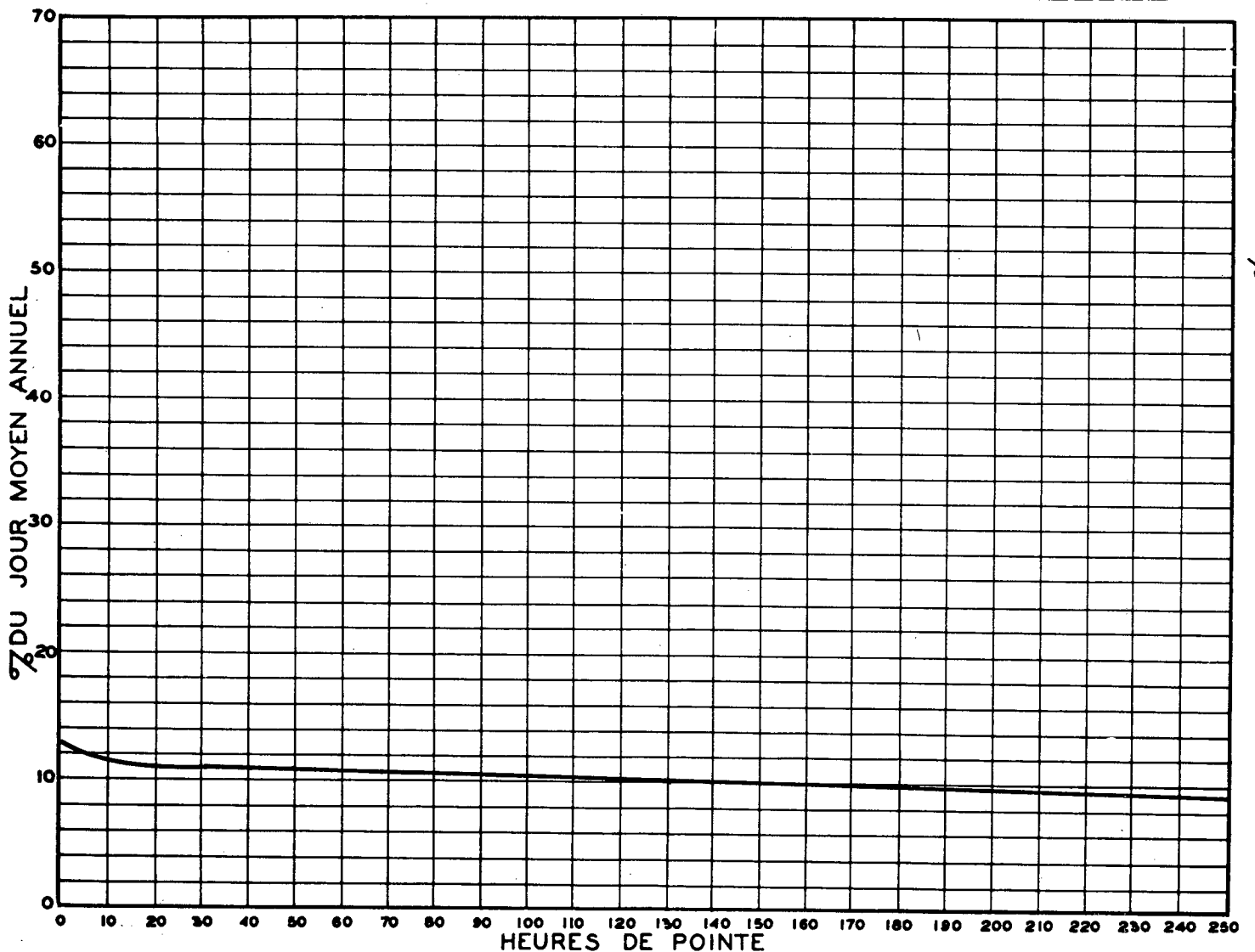
RELATION ENTRE LES HEURES DE POINTE ET LE JOUR MOYEN ANNUEL STATION: ST-NICOLAS 2 VOIES ROUTE N° RS-32-199
