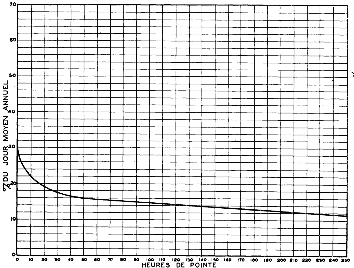
RELATION ENTRE LES HEURES DE POINTE ET LE JOUR MOYEN ANNUEL STATION: ST-GREGOIRE ROUTE N° 3-4-5
