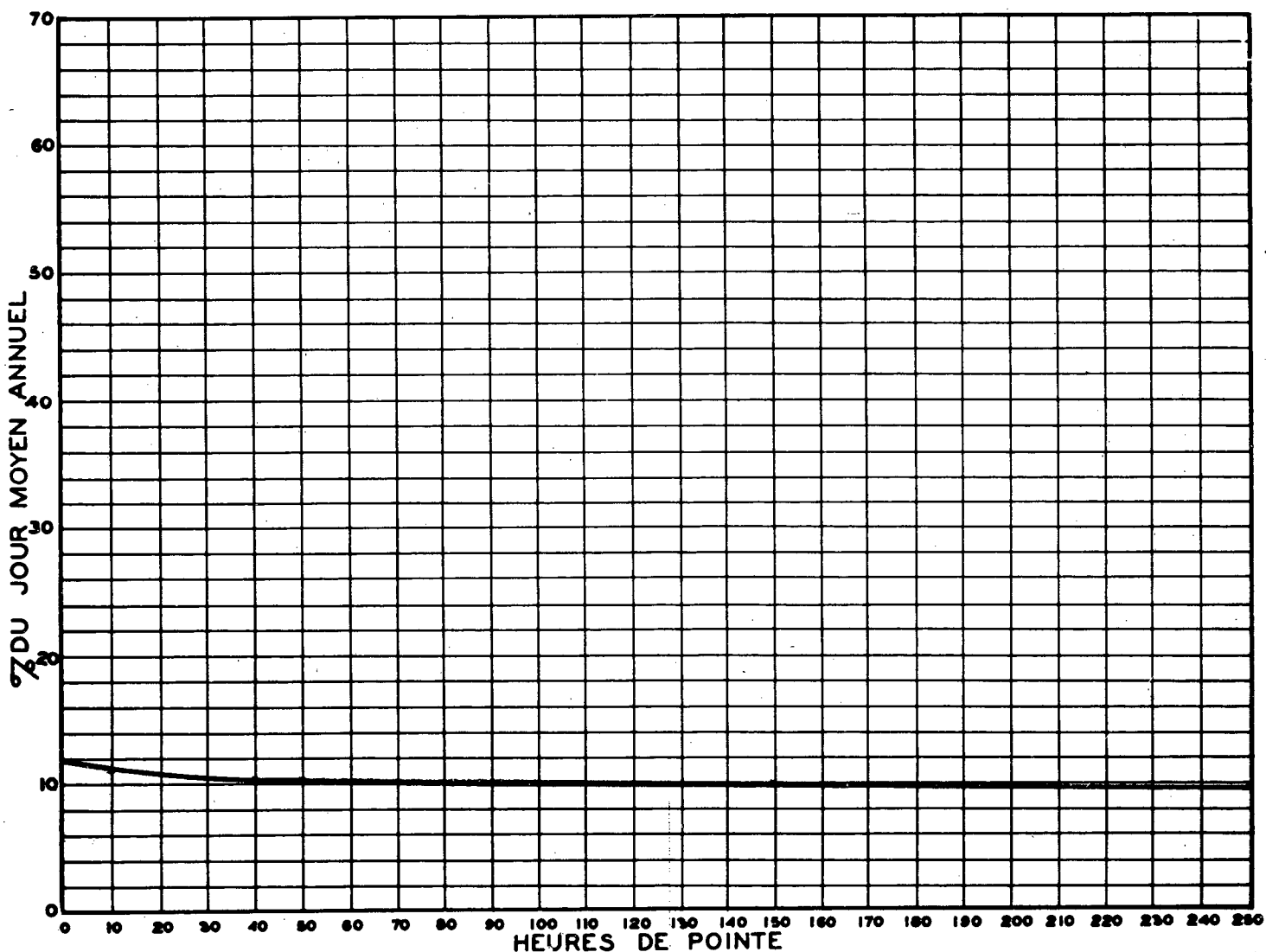
RELATION ENTRE LES HEURES DE POINTE ET LE JOUR MOYEN ANNUEL STATION: DORVAL 2 VOIES ROUTE N° 20-63-752
