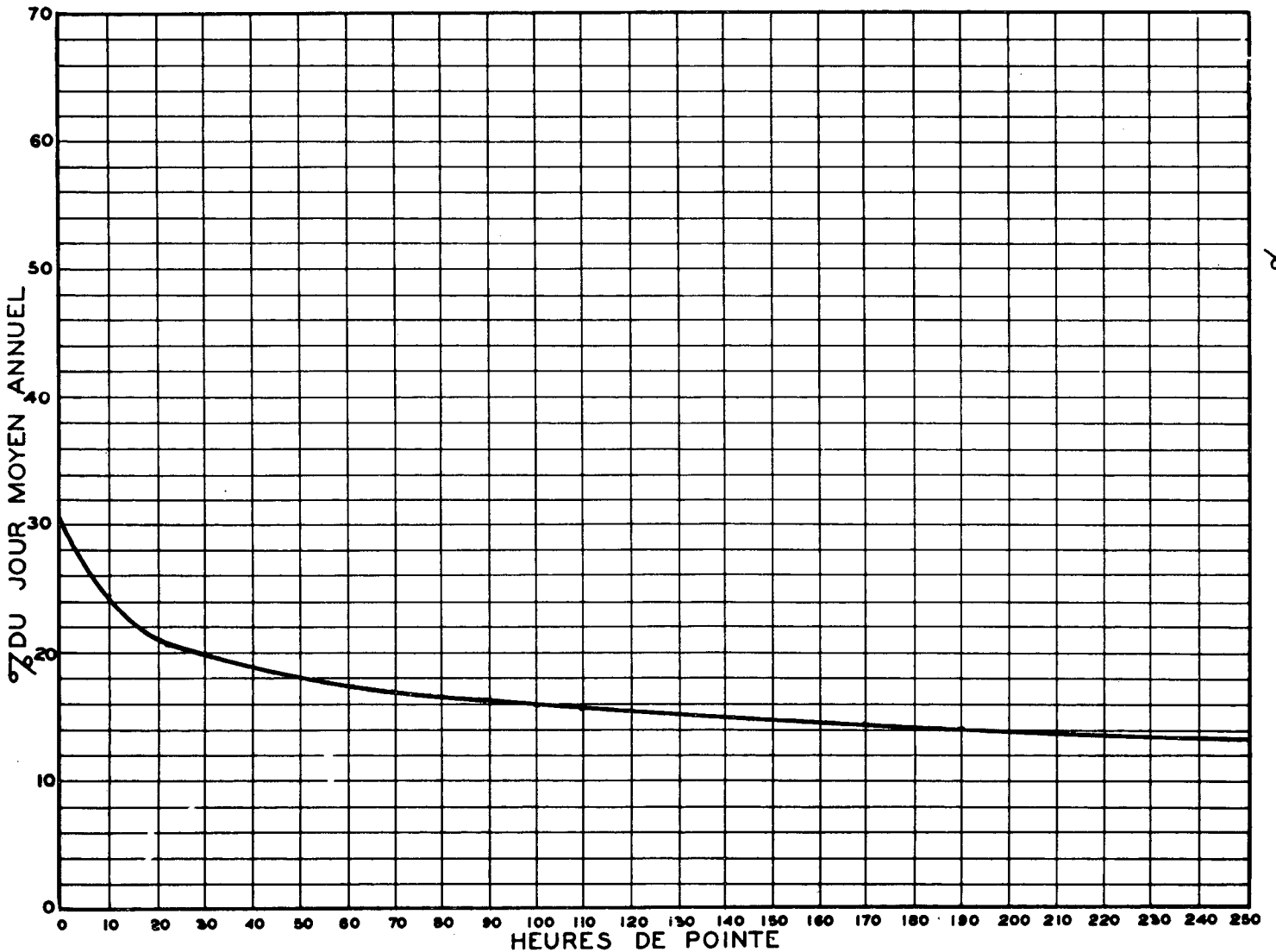
RELATION ENTRE LES HEURES DE POINTE ET LE JOUR MOYEN ANNUEL STATION: BERTHIER VOIE NORD ROUTE N° 20-32-223
