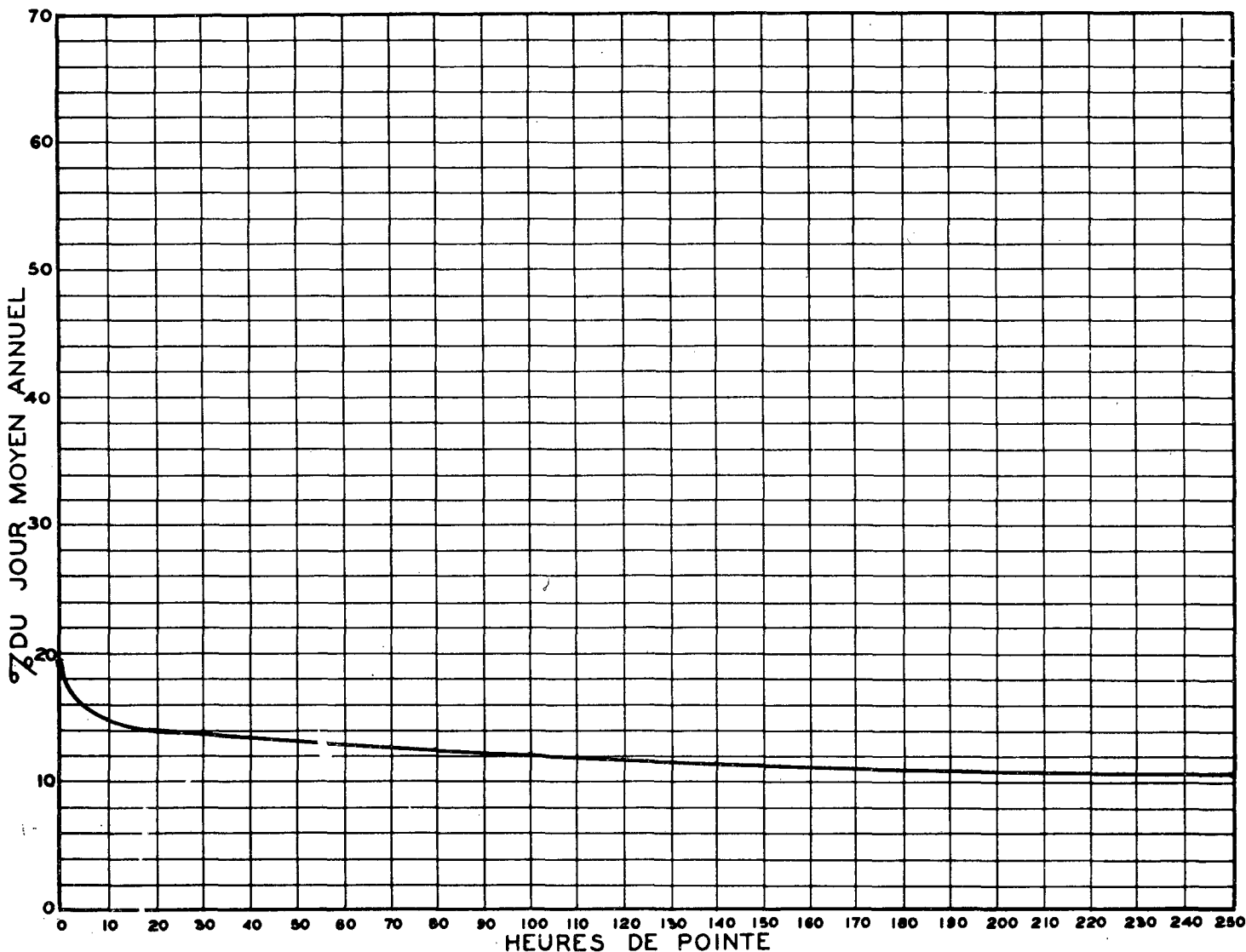
RELATION ENTRE LES HEURES DE POINTE ET LE JOUR MOYEN ANNUEL STATION: ST-BERNARD ROUTE N° 1-32-1
