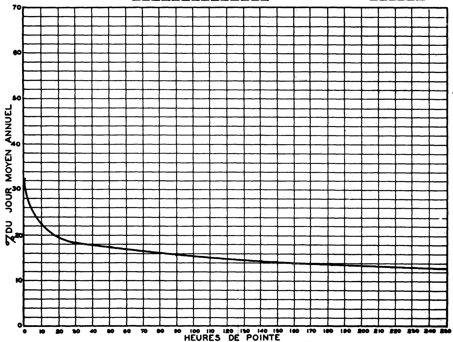
RELATION ENTRE LES HEURES DE POINTE ET LE JOUR MOYEN ANNUEL STATION: BERTHIER VOIE SUD ROUTE N° 20-32-223
