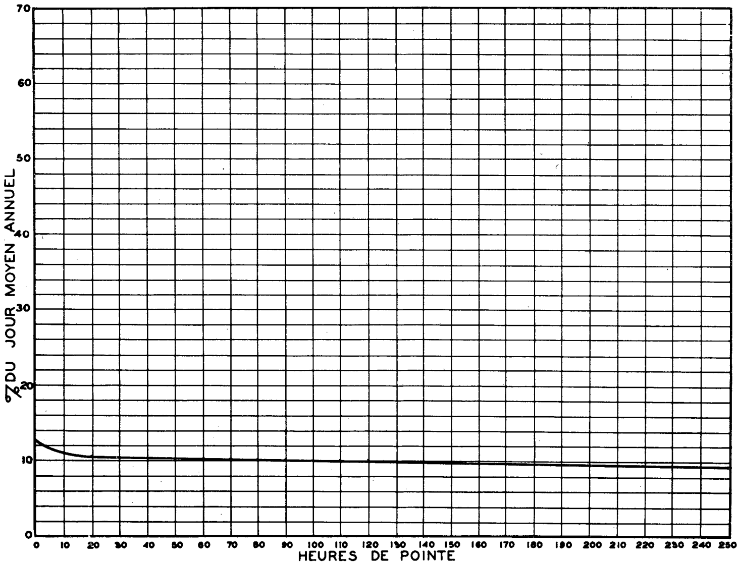
RELATION ENTRE LES HEURES DE POINTE ET LE JOUR MOYEN ANNUEL — STATION: SILLERY ROUTE N° RS-31-169
