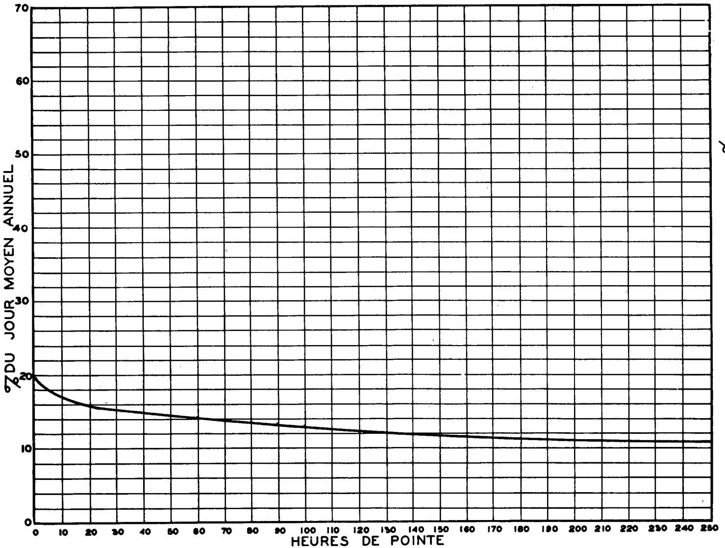
RELATION ENTRE LES HEURES DE POINTE ET LE JOUR MOYEN ANNUEL STATION: ST-ETIENNE ROUTE N° 5-32-7
