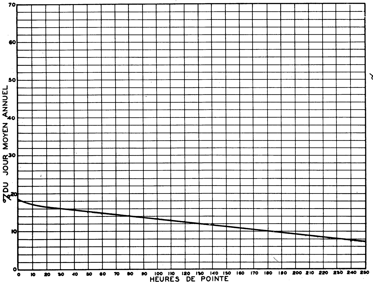
RELATION ENTRE LES HEURES DE POINTE ET LE JOUR MOYEN ANNUEL STATION: LONGUEUIL VOIE NORD ROUTE N° 9-62-80
