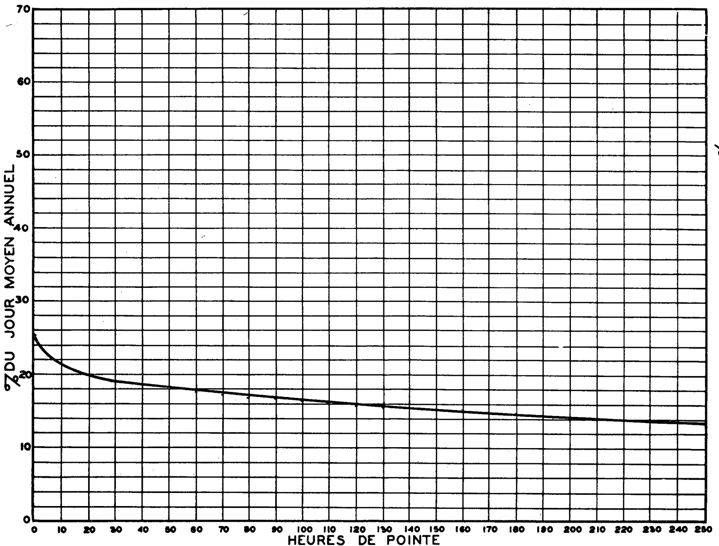
RELATION ENTRE LES HEURES DE POINTE ET LE JOUR MOYEN ANNUEL — STATION: STE-FÉLICITE ROUTE N° 6-1-1
