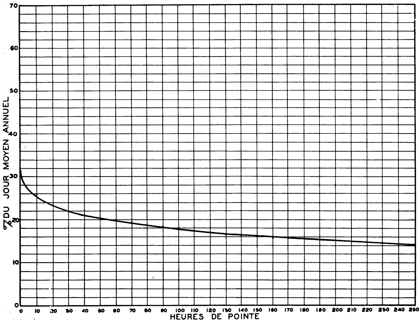
RELATION ENTRE LES HEURES DE POINTE ET LE JOUR MOYEN ANNUEL STATION: BERTHIER ROUTE N° 2-32-3
