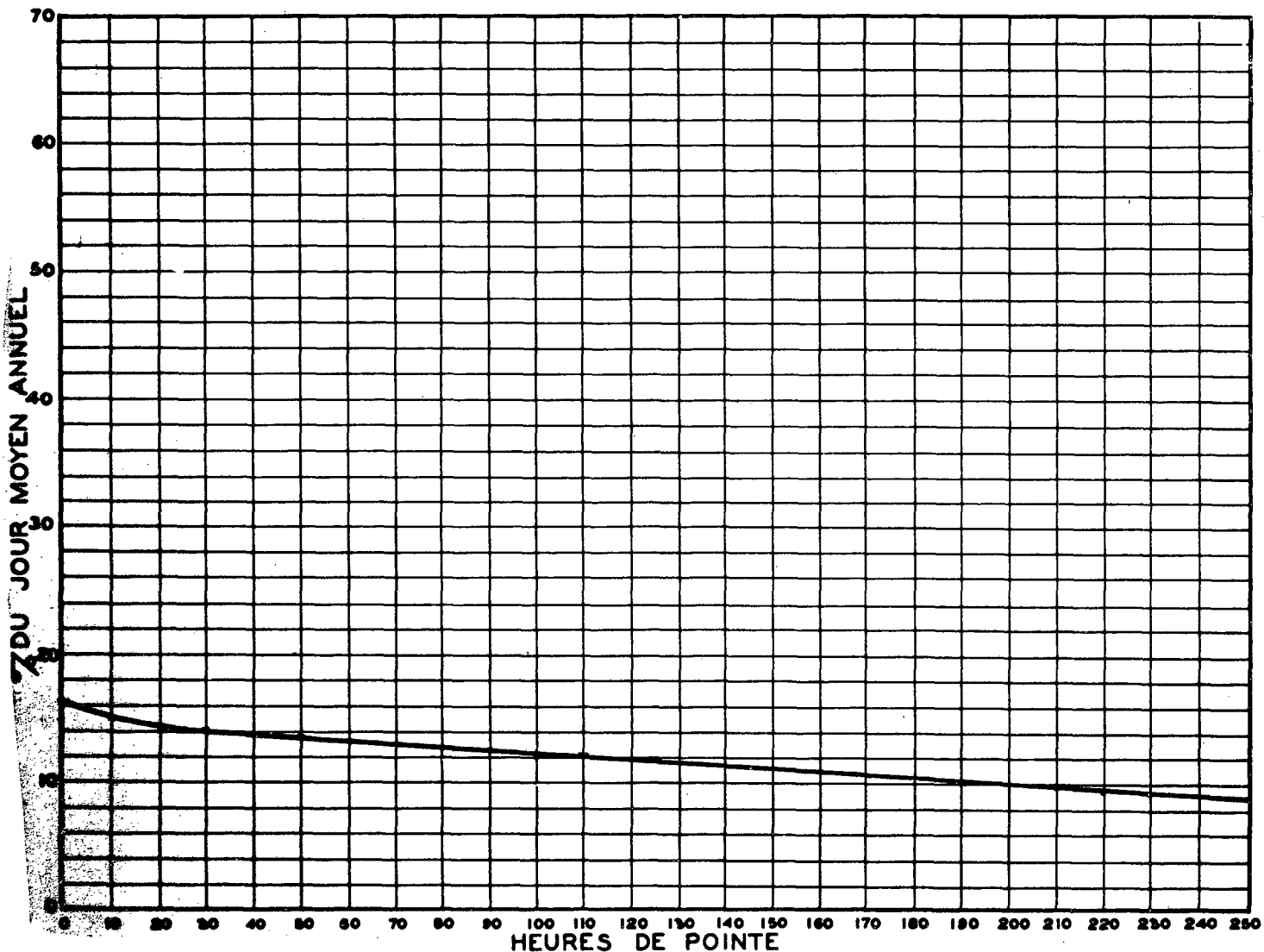
RELATION ENTRE LES HEURES DE POINTE ET LE JOUR MOYEN ANNUEL STATION: VILLE-MARIE VOIE NORD ROUTE N° 20-63-734
