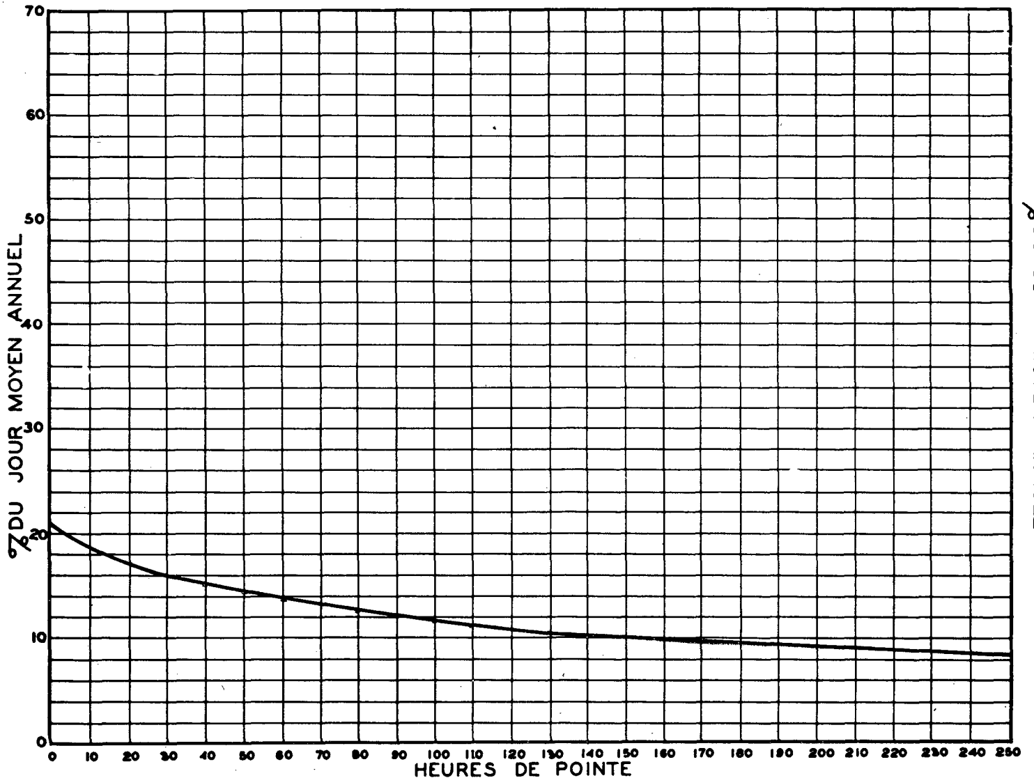
RELATION ENTRE LES HEURES DE POINTE ET LE JOUR MOYEN ANNUEL STATION: SABREVOIS ROUTE N° 7-62-64
