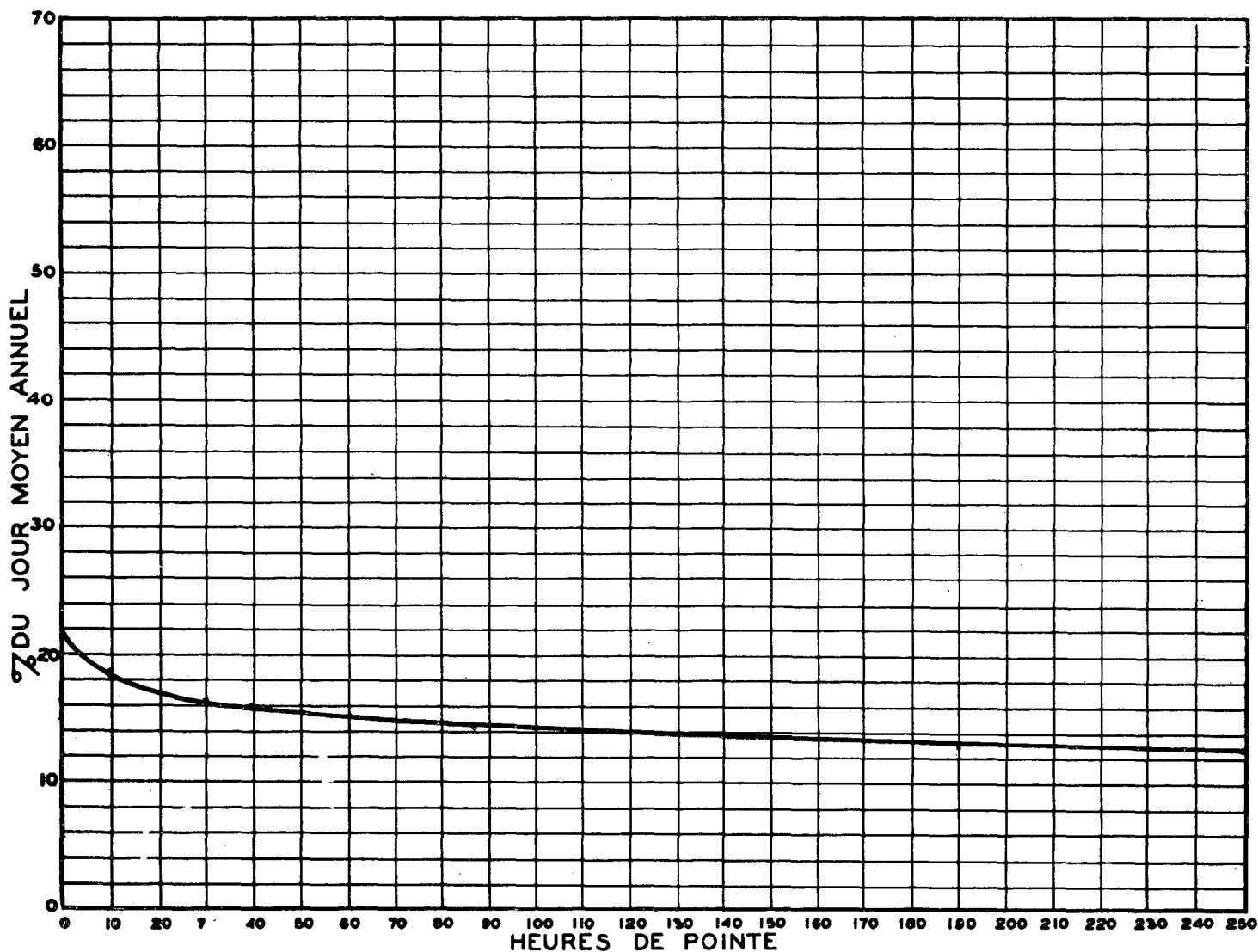
RELATION ENTRE LES HEURES DE POINTE ET LE JOUR MOYEN ANNUEL STATION: BERTHIER 2 VOIES ROUTE N° 20-32-223
