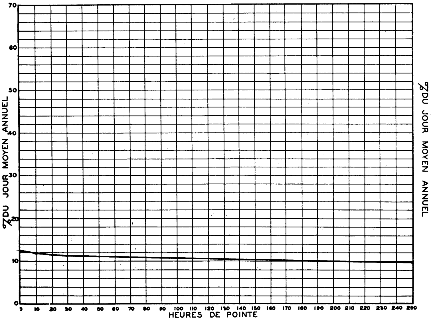
RELATION ENTRE LES HEURES DE POINTE ET LE JOUR MOYEN ANNUEL STATION: MONTREAL 2 VOIES ROUTE N° RS-63-504
