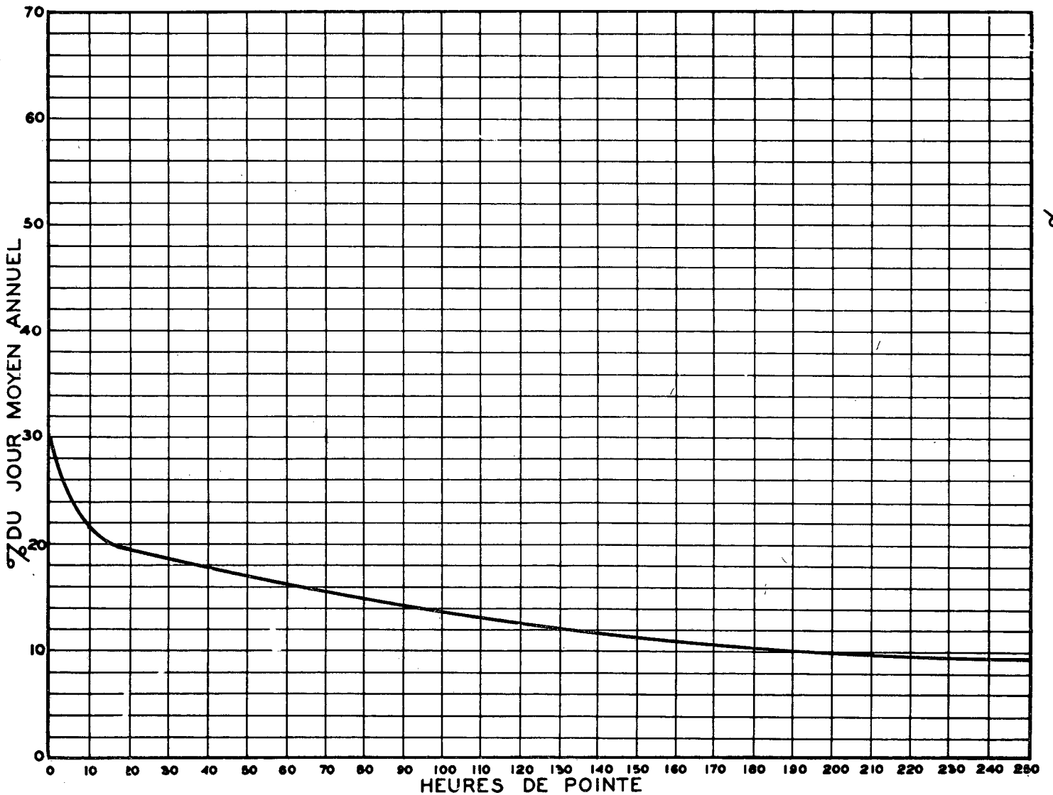
RELATION ENTRE LES HEURES DE POINTE ET LE JOUR MOYEN ANNUEL STATION: VAUDREUIL VOIE SUD ROUTE N° 20-63-802
