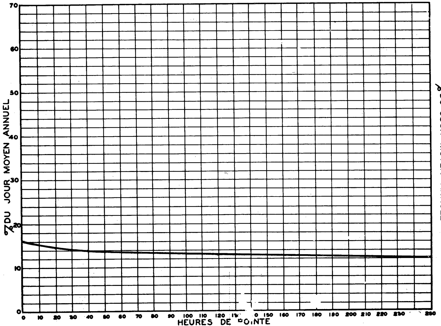
RELATION ENTRE LES HEURES DE POINTE ET LE JOUR MOYEN ANNUEL — STATION: PONT GALIPEAULT VOIE NORD — — — — — ROUTE N° 20-63-802 — — — — —
