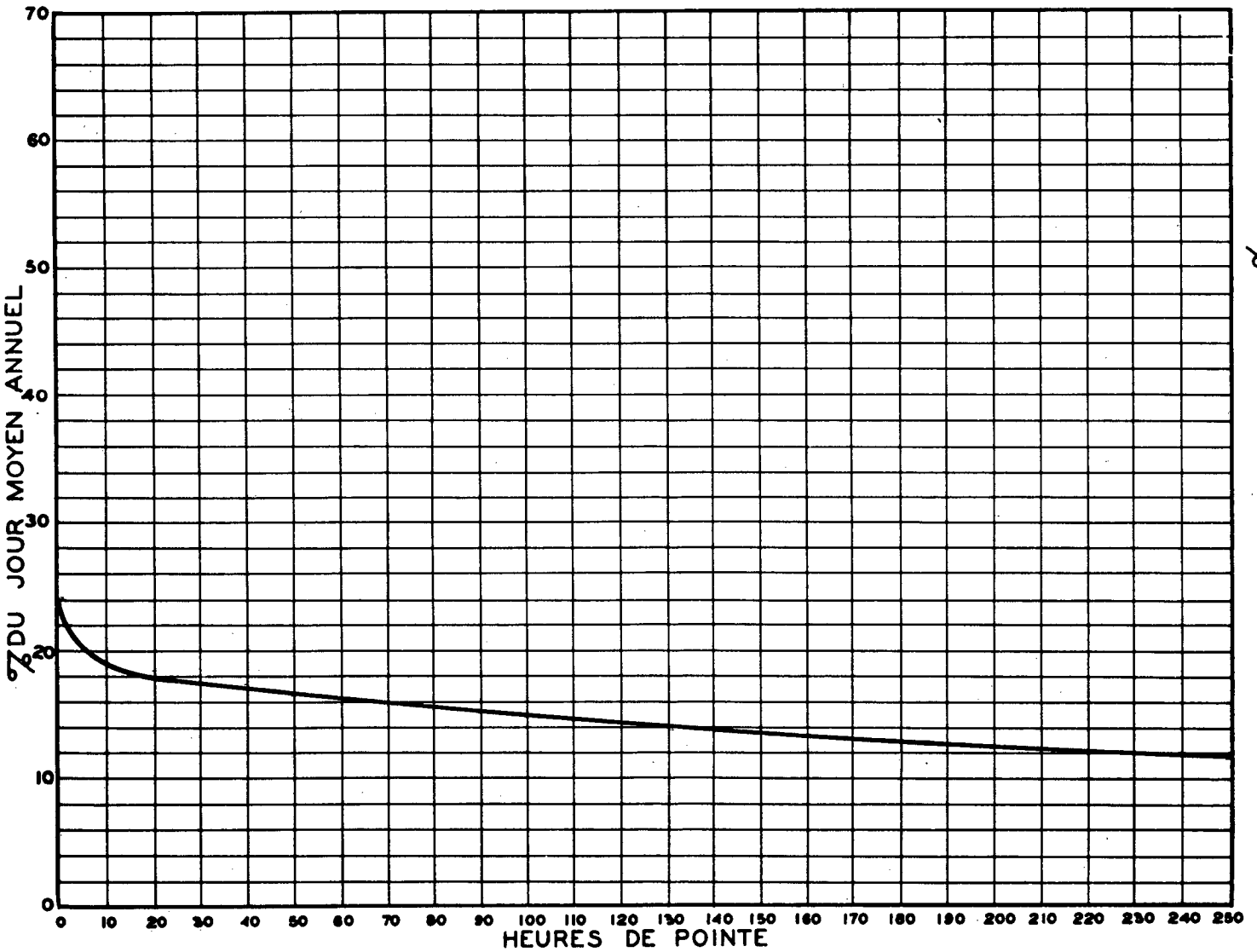
RELATION ENTRE LES HEURES DE POINTE ET LE JOUR MOYEN ANNUEL — STATION: ST-BLAISE ROUTE N° 223-62-85
