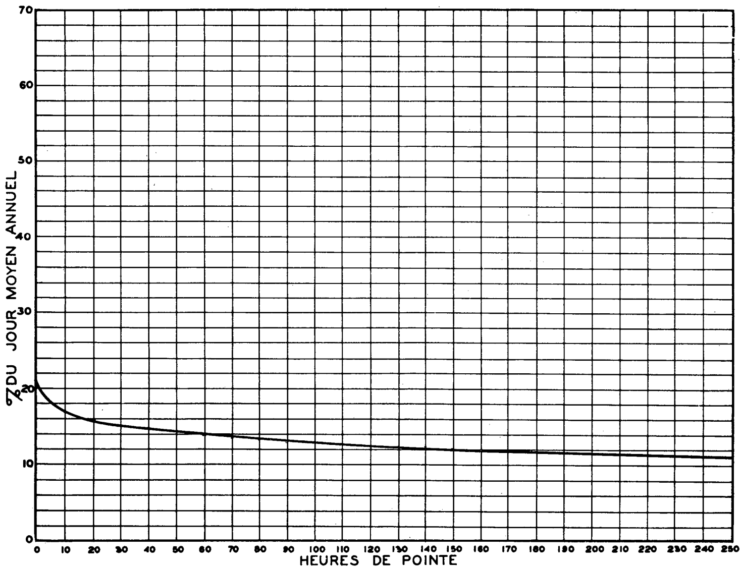
RELATION ENTRE LES HEURES DE POINTE ET LE JOUR MOYEN ANNUEL STATION: DESCHAMBAULT ROUTE N° 2-31-8
