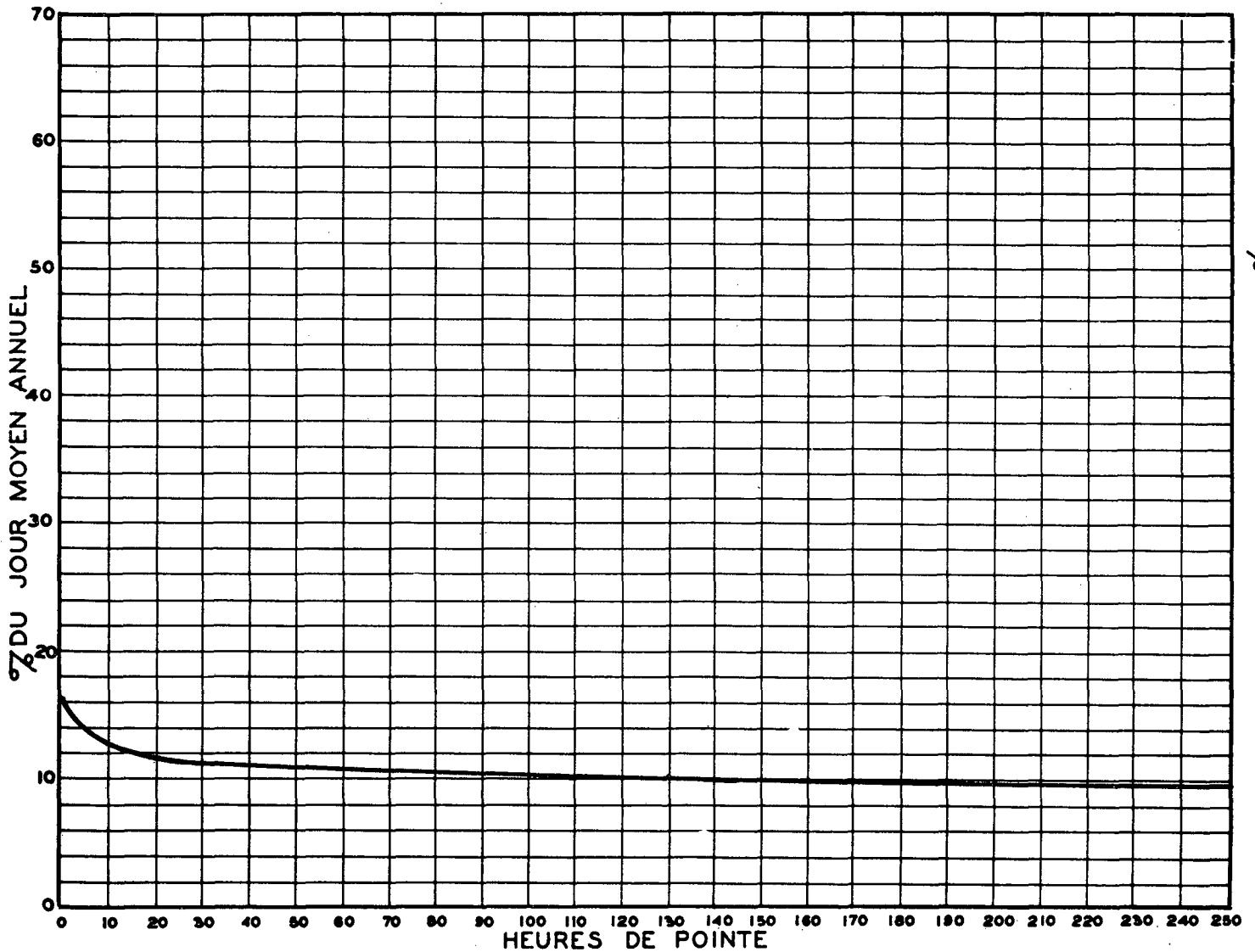
RELATION ENTRE LES HEURES DE POINTE ET LE JOUR MOYEN ANNUEL — STATION: TERREBONNE ROUTE N° 18-64-70
