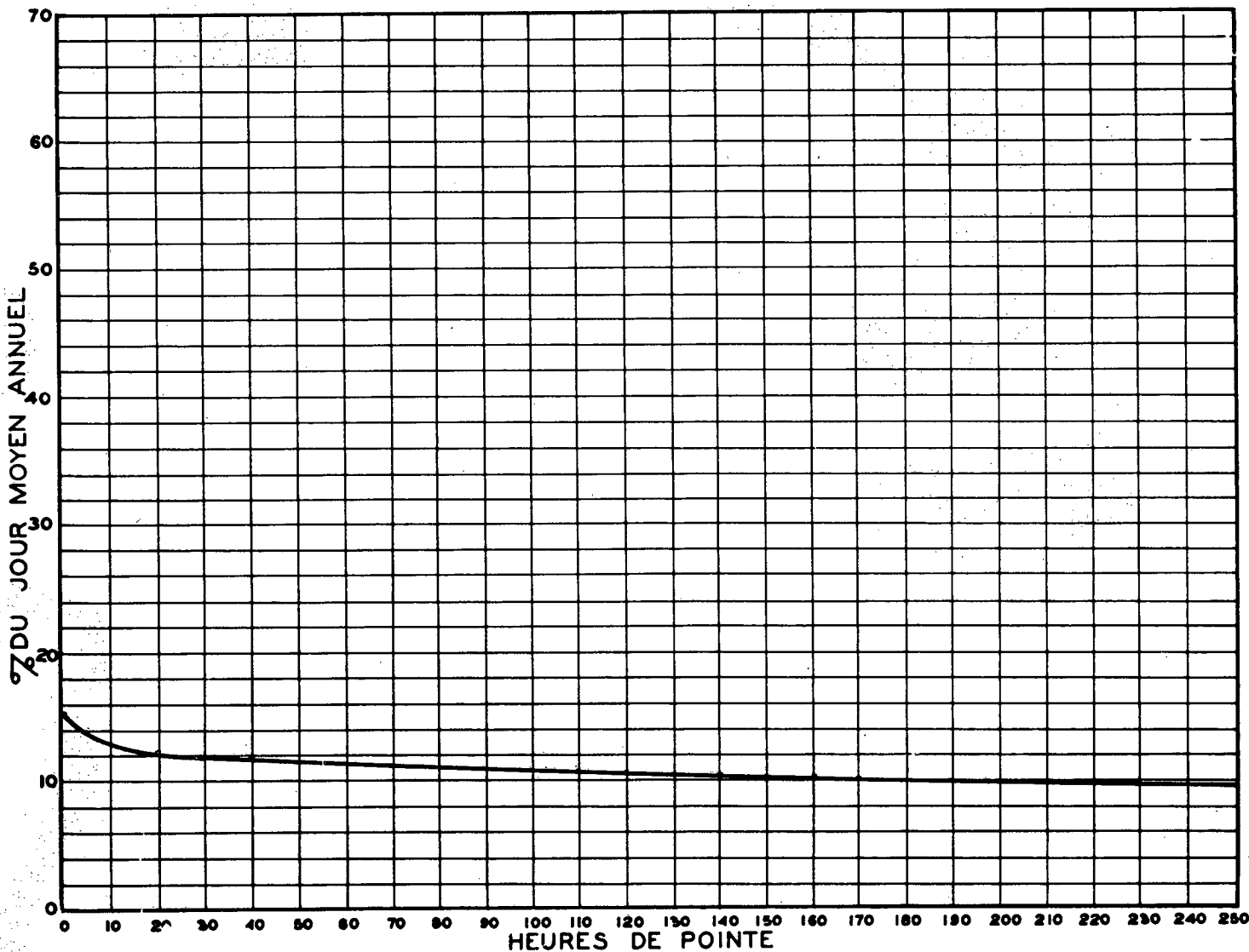
RELATION ENTRE LES HEURES DE POINTE ET LE JOUR MOYEN ANNUEL STATION: LENNOXVILLE ROUTE N° 5-5-11
