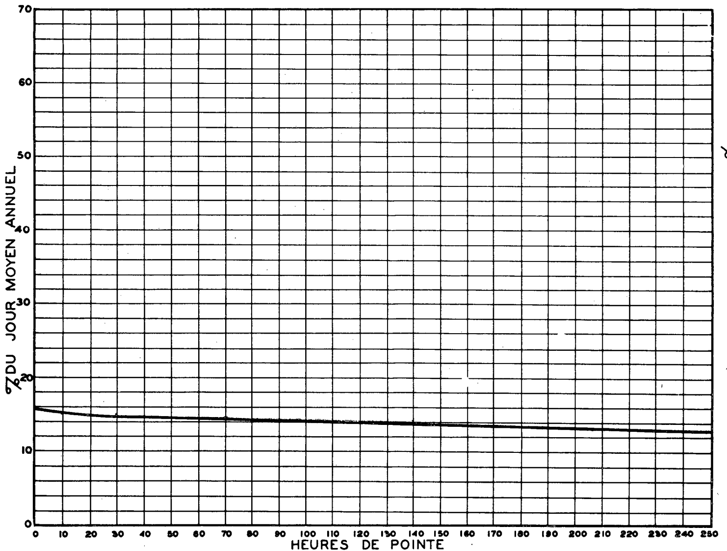
RELATION ENTRE LES HEURES DE POINTE ET LE JOUR MOYEN ANNUEL STATION: PONT MERCIER VOIE EST ROUTE N° 4-63-83
