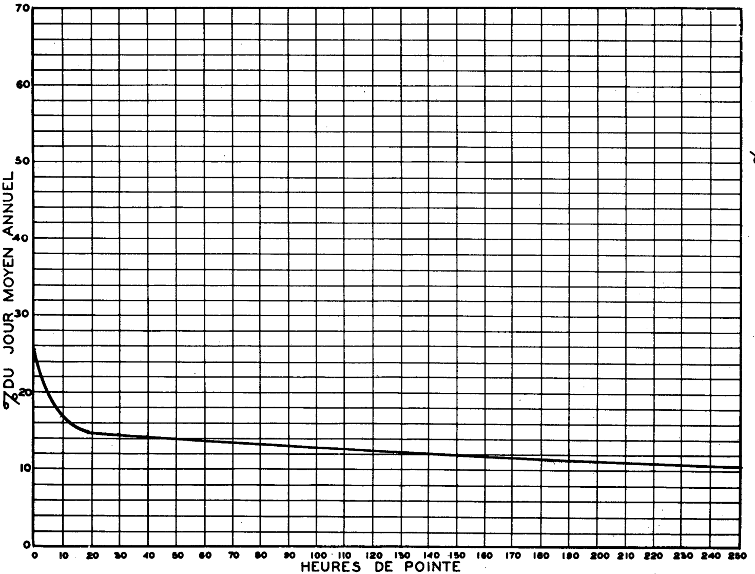
RELATION ENTRE LES HEURES DE POINTE ET LE JOUR MOYEN ANNUEL — STATION: CHAMBORD ROUTE N° 169-2-380
