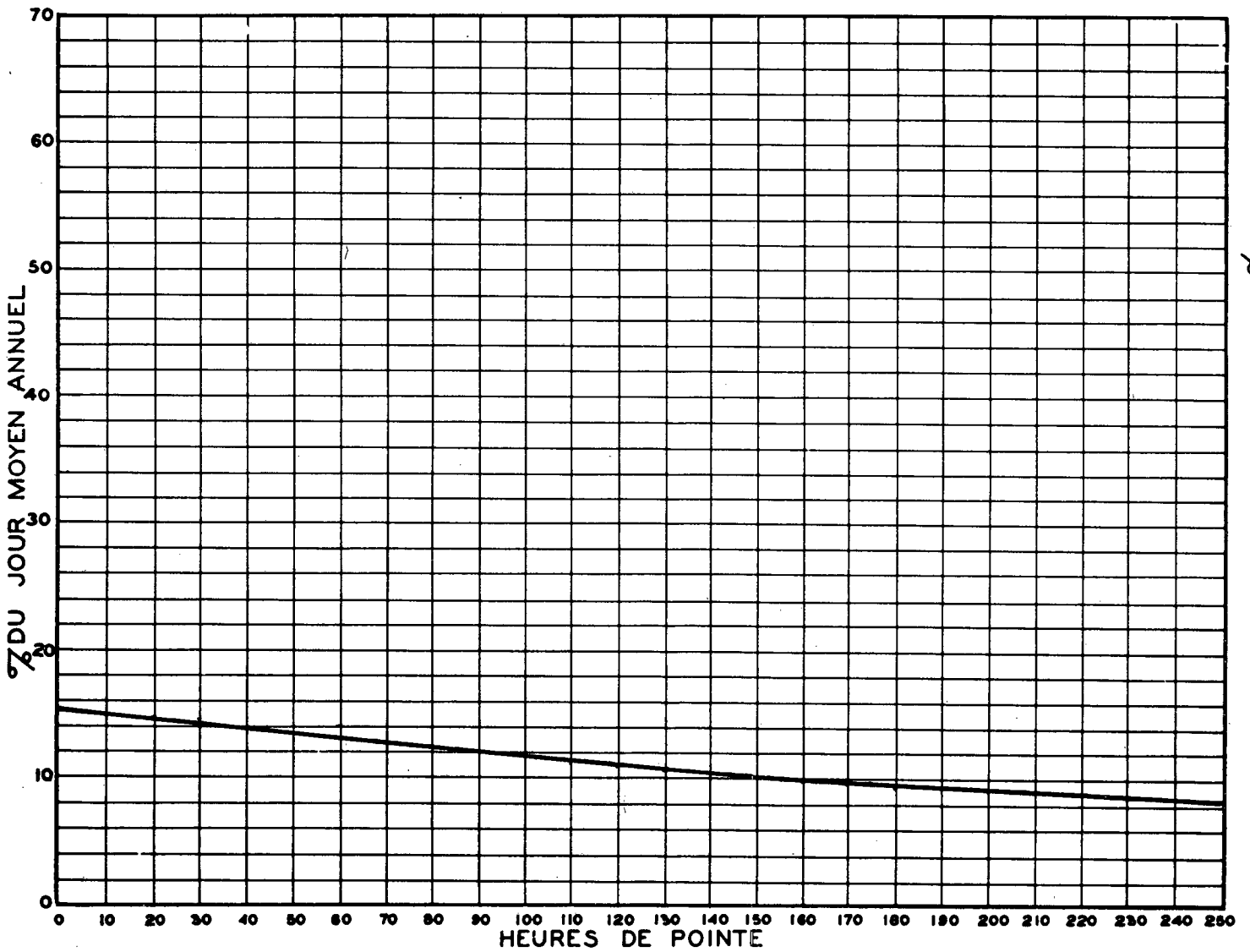
RELATION ENTRE LES HEURES DE POINTE ET LE JOUR MOYEN ANNUEL STATION: PONT MERCIER VOIE OUEST ROUTE N° 4-63-83
