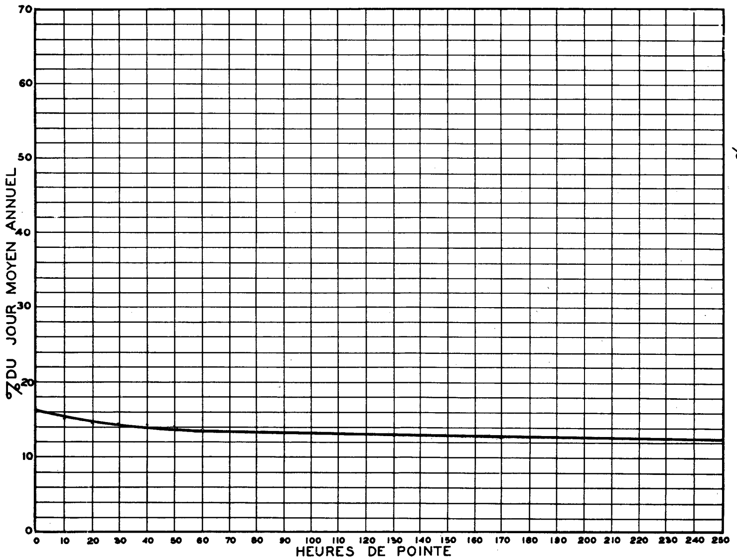
RELATION ENTRE LES HEURES DE POINTE ET LE JOUR MOYEN ANNUEL STATION: POINTE AUX TREMBLES VOIE EST ROUTE N° 2-63-85
