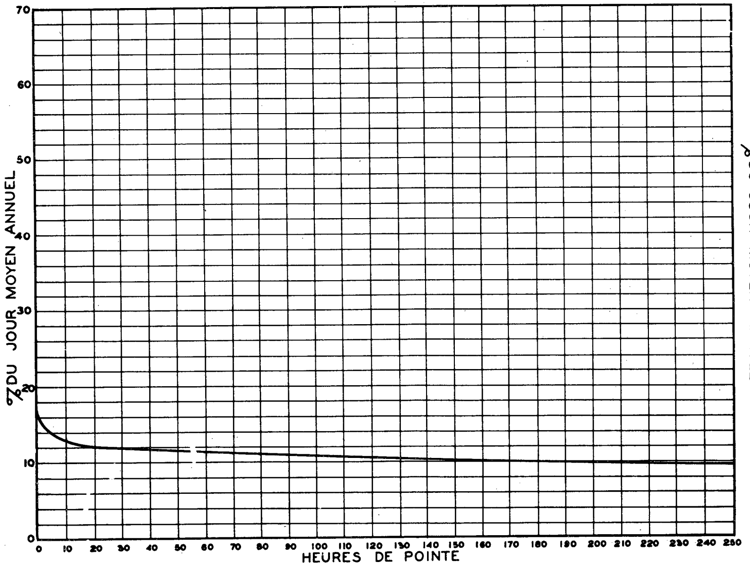
RELATION ENTRE LES HEURES DE POINTE ET LE JOUR MOYEN ANNUEL — STATION: MAGOG VOIE SUD ROUTE N° 1-5-3
