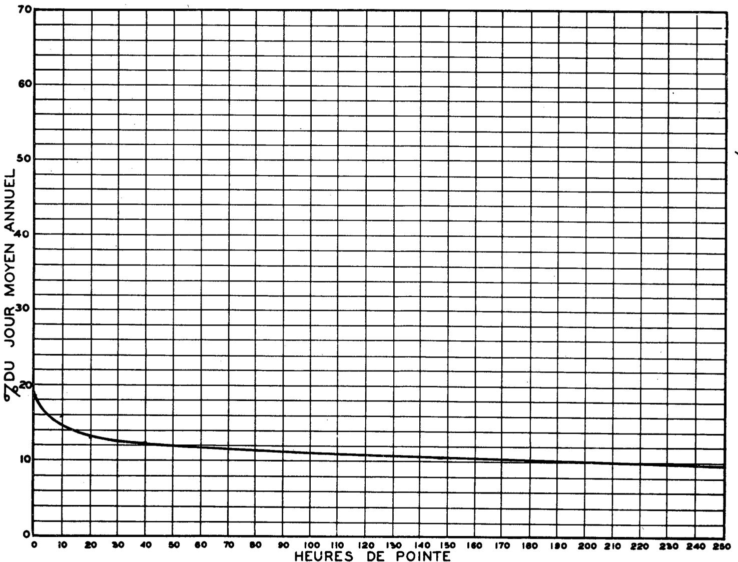
RELATION ENTRE LES HEURES DE POINTE ET LE JOUR MOYEN ANNUEL STATION: VAUDREUIL 2 VOIES ROUTE N° 40-63-802
