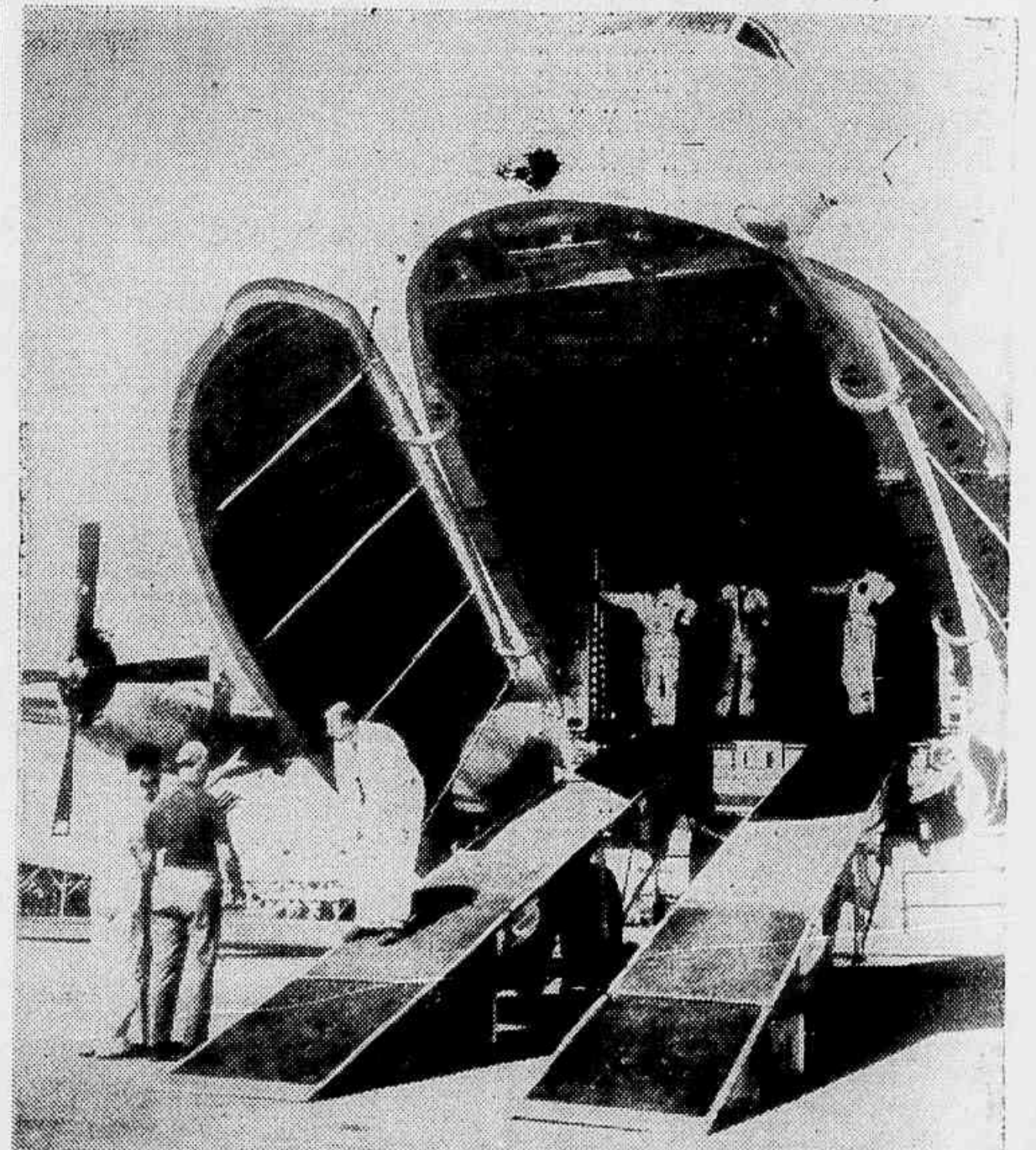
A fotografia ilustra o Douglas C-124, Globemaster II, avião transporte da Força Aérea dos Estados Unidos, mostrando o funcionamento do novo sistema de portas, para o compartimento de carga e descarga, sendo-se ainda as rampas escamoteáveis, para facilidade de manobra. (USIS)
