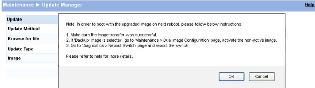
Figure 10-8. Update Steps
